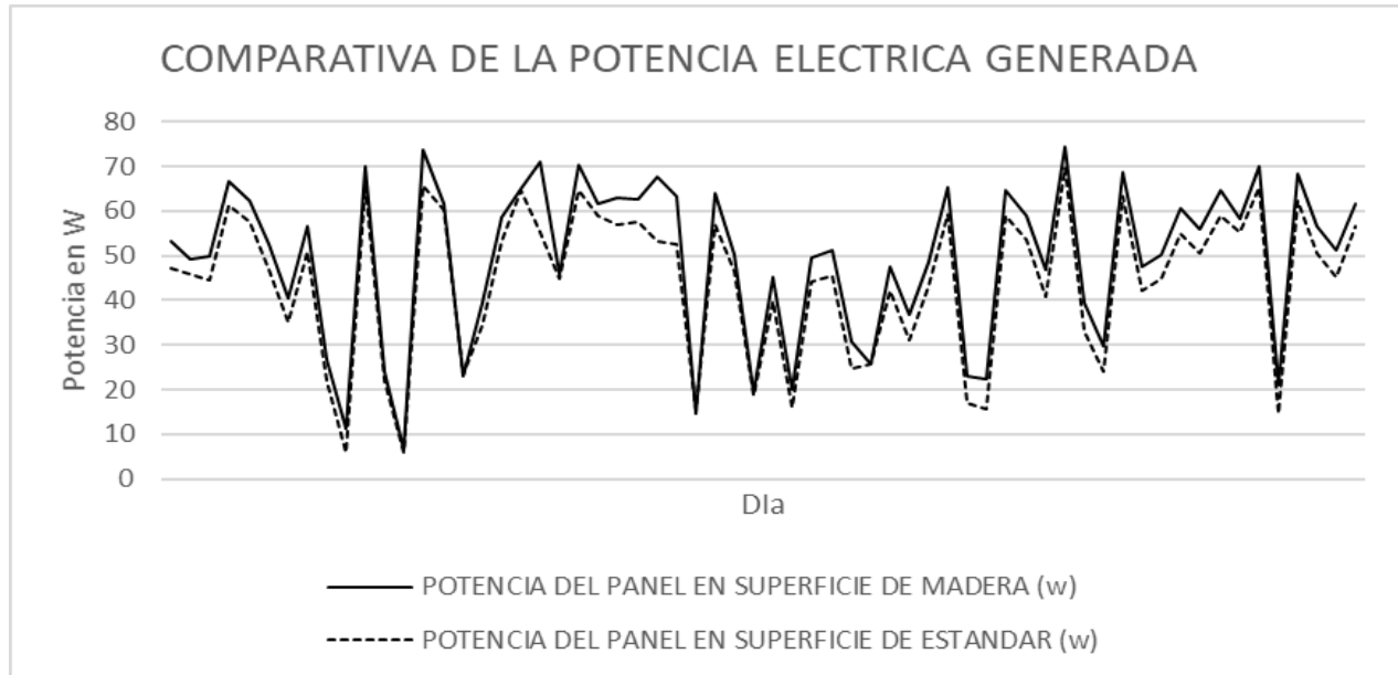
Gráfico 4 Comparativa de la potencia eléctrica generada. (Datos recolectados 12:00 m)
