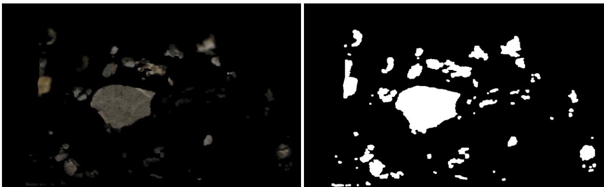
Figura 16. Segmentación mezcla MF-40
