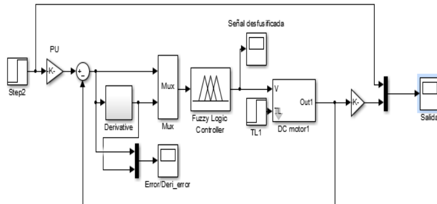
Figura 7 Diagrama de bloques controlador difuso.
