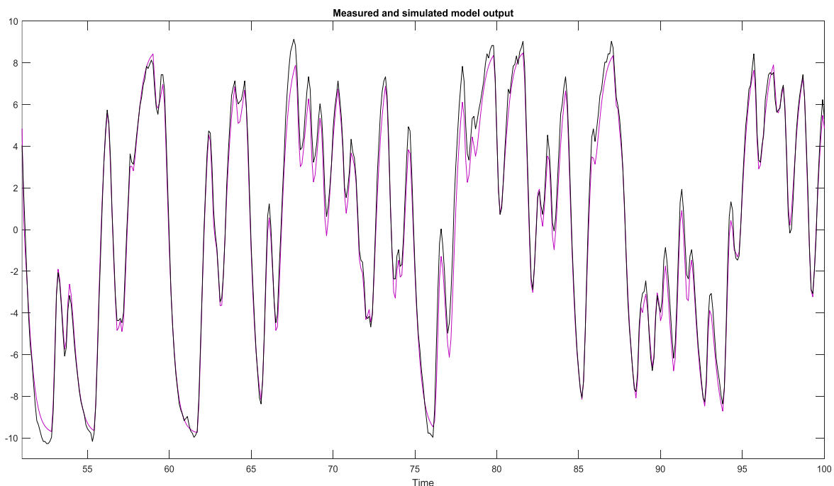
Figura 7. Adaptación de la red NN-NARX a los datos de temperatura. Fuente: elaboración propia
