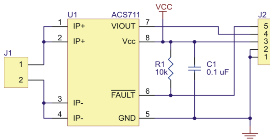
Figura 15 Esquema sensor de corriente
