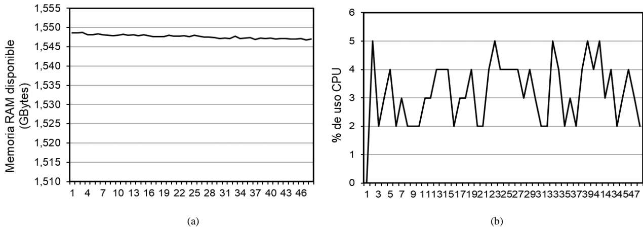
Figura 10. Medidas de desempeño del gateway: (a) Memoria RAM disponible y (b) Porcentaje de uso de la CPU
