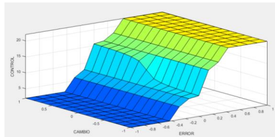
Figura 5 Superficie de control.
