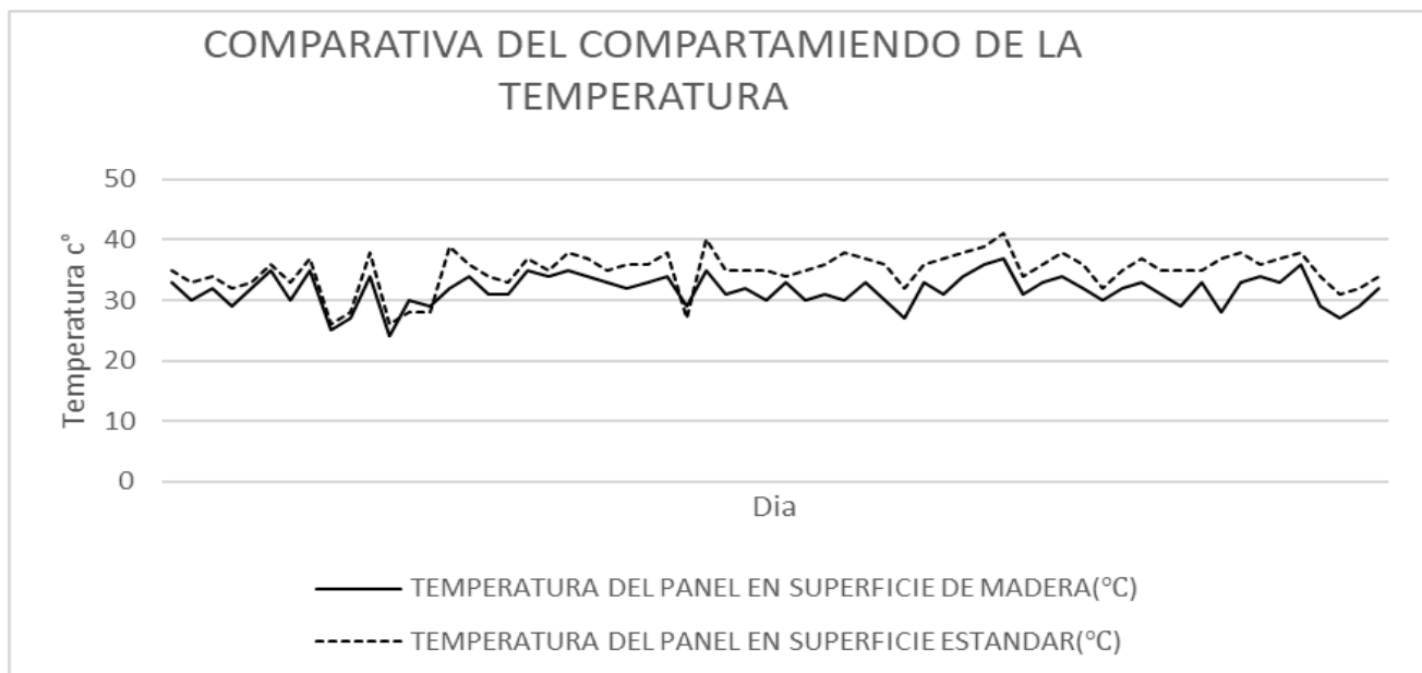
Gráfico 1 Comparativa del comportamiento de la temperatura (Datos recolectados 8:00 am) Fuente: elaboración propia de los autores.
