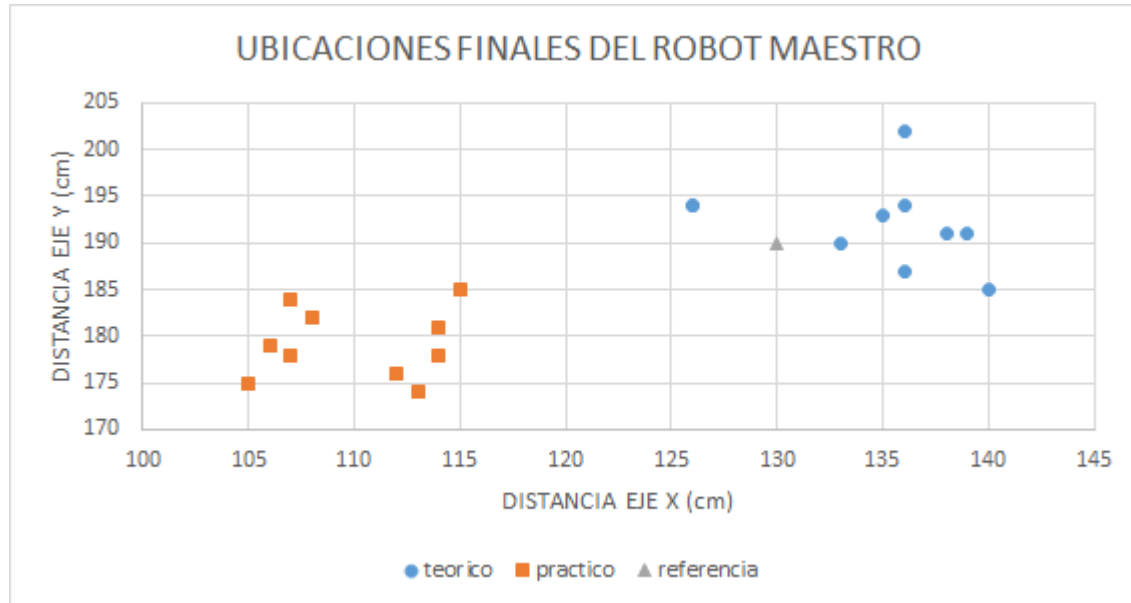
Figura 13. Ubicación final robot maestro para la coordenada deseada x = 130 , y = 190 . (fuente de elaboración propia)
