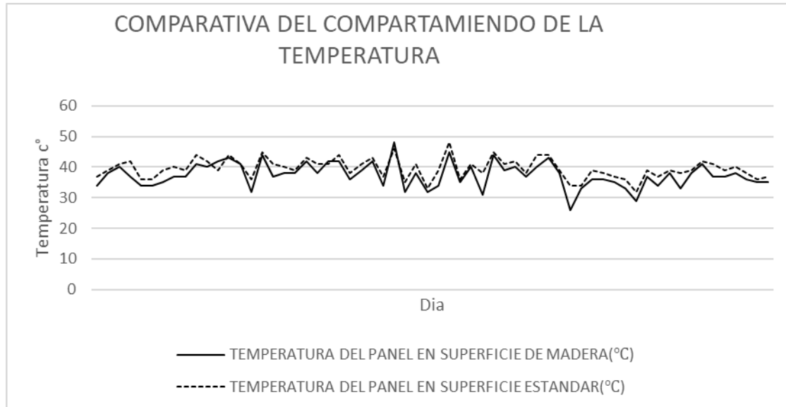
Gráfico 3 Comparativa de la temperatura (Datos recolectados 12:00 am) Fuente: elaboración propia de los autores.
