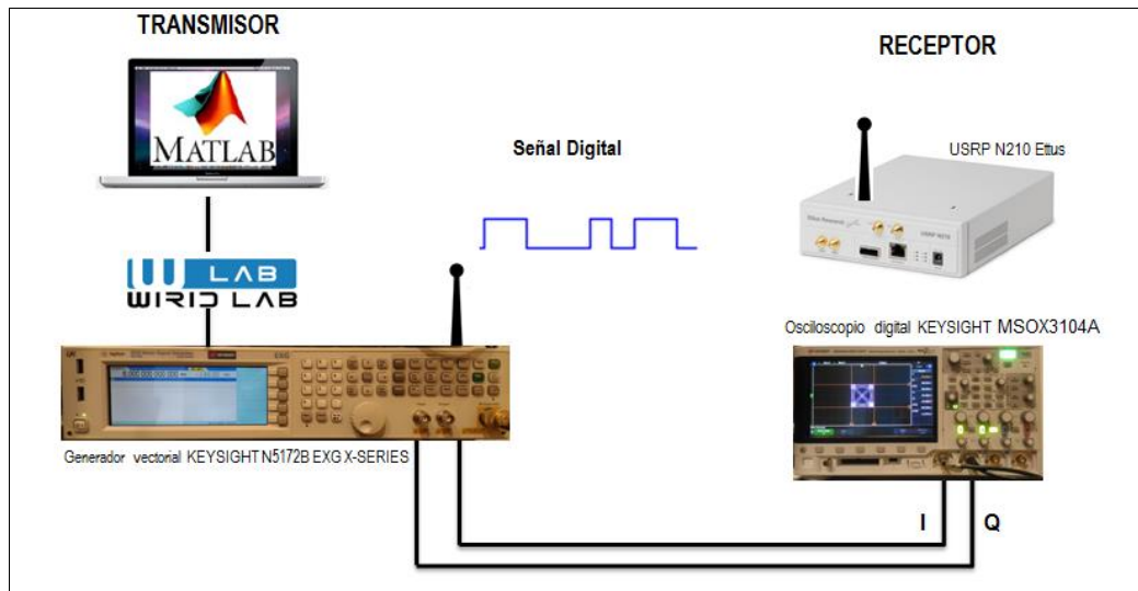
Figura 11. Esquema implementación modulaciónes usando MATLAB.
