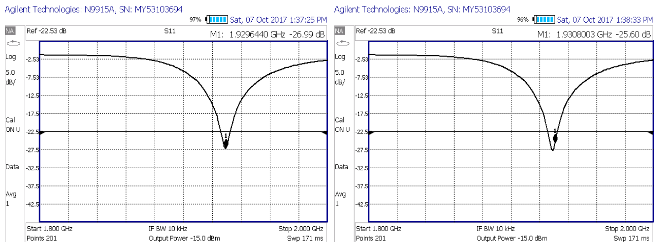
Figura 16(a). Medición del parámetro S11 magnitud en dB del segundo diseño de antena. (b) Medición del parámetro S11 magnitud en dB del segundo diseño de antena con marcador en la frecuencia deseada Fuente: Analizador Vectorial Keysight N9915A
