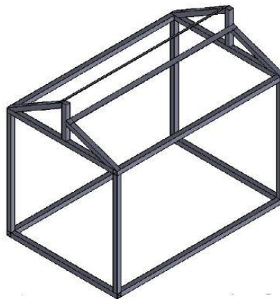
Figura 10. Diseño estructural. Fuente: Elaboración propia
