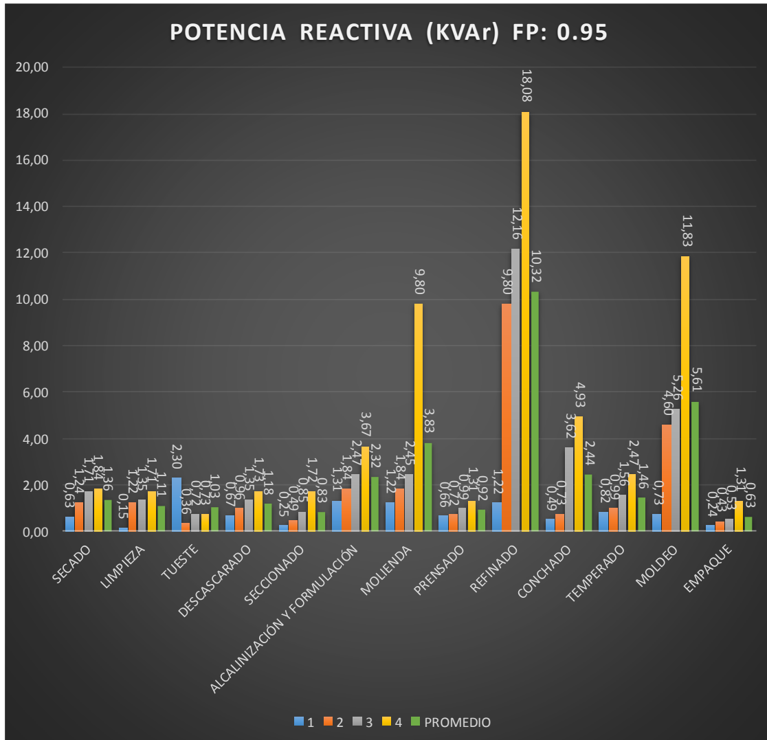
Figura 6. Potencia Reactiva para un Factor de Potencia de 0,95
