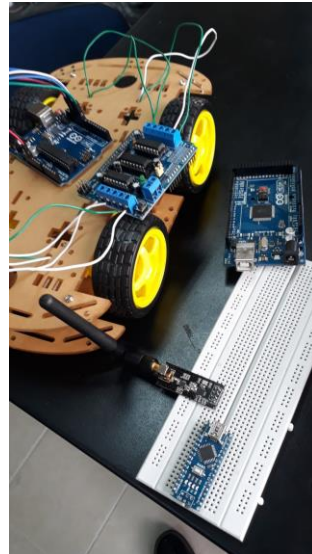
Figura 10. Sistema de control de carro – robot. Fuente: elaboración propia de los autores.
