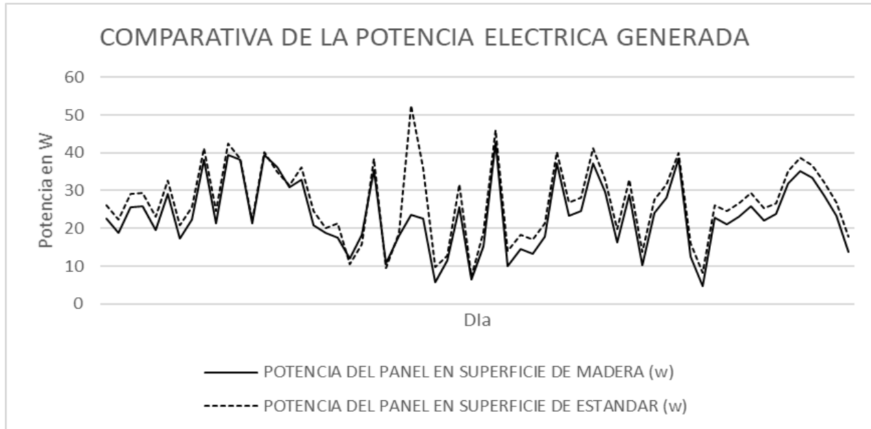
Gráfico 2 Comparativa de la potencia eléctrica generada. (Datos recolectados 8:00 am)
