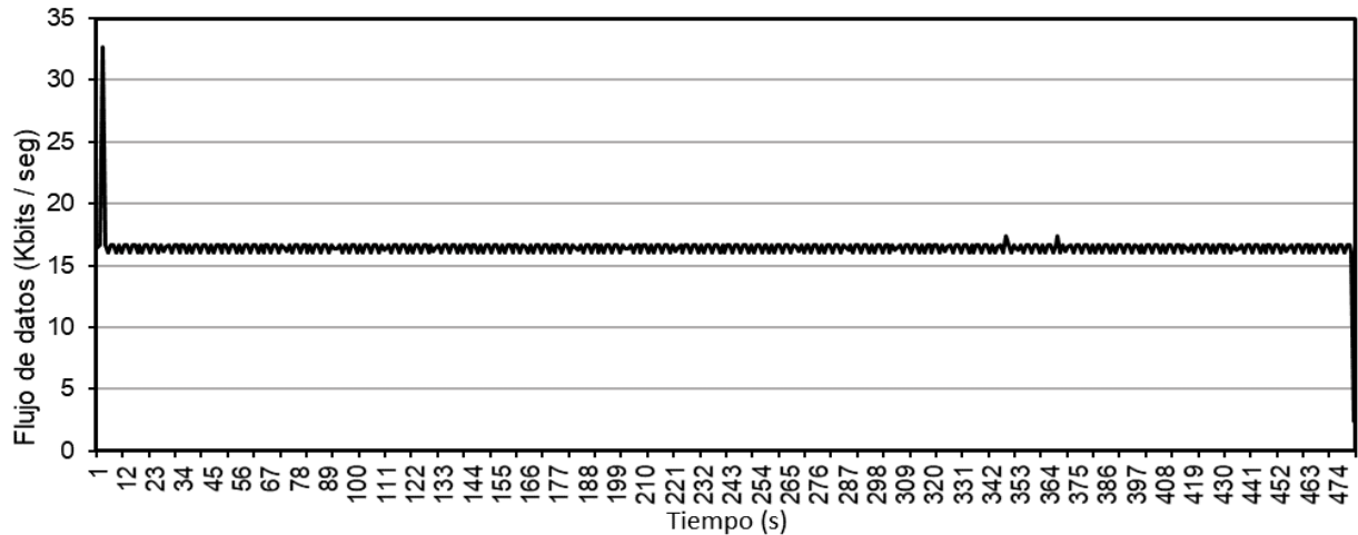
Figura 9. Tráfico recibido a través de ZigBee
