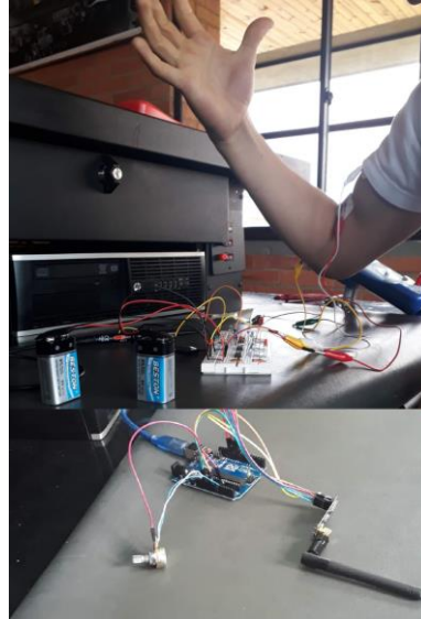
Figura 10. Modo de transmisión de la señal EMG. Fuente: Elaboración Propia de los autores
