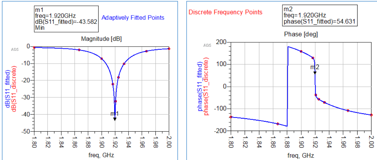
Figura 9. Resultado de la sintonización de \epsilon_r con ADS Fuente: ADS Software
