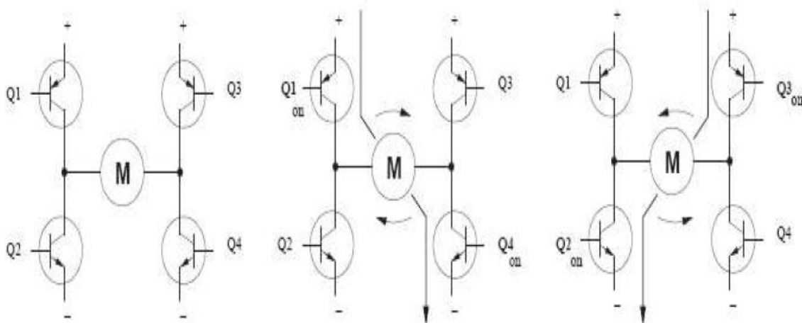
Figura 10 Representación Puente H
