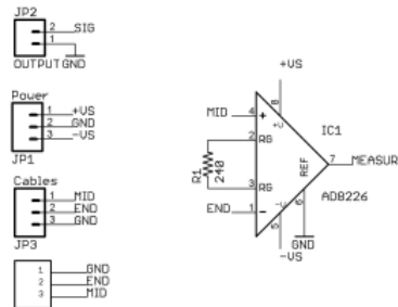
Figura 4. Circuito de la etapa amplificadora. Fuente: Brian Kaminski ARA/SED, 2014, "Muscle sensor V3", Recuperado de: http://www.advancertechnologies.com/p/muscle-sensor-v3.html .
