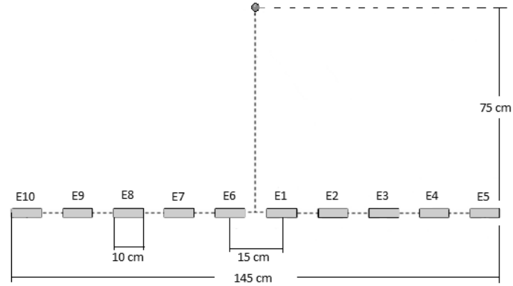
Figura 2. Distancias entre reflectores primarias. Fuente: elaborado por autores
