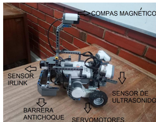
Figura 1. Robot maestro. (fuente de elaboración propia)
