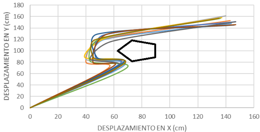
Figura 14. Recorrido del convoy para una coordenada final en x = 140 , y = 150 con obstáculo. (fuente de elaboración propia)
