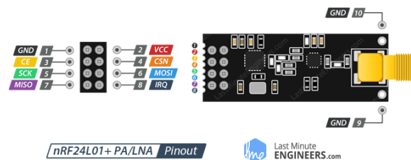
Figura 9. Se muestra el diagrama de pines de la Antena NRF24L01. Fuente: Patagoniatec, “NRF24L01 + RFX2401”, 2014, Recuperado de: https://saber.patagoniatec.com/2014/07/nrf24l01-rfx2401-nrf24l01-pa-lna-arduino-argentina-ptec/ .
