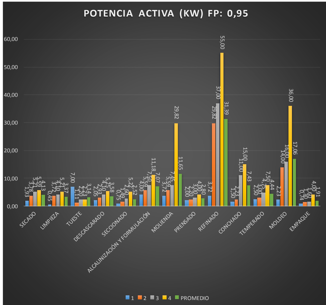
Figura 2 Potencia Activa para un Factor de Potencia de 0,95
