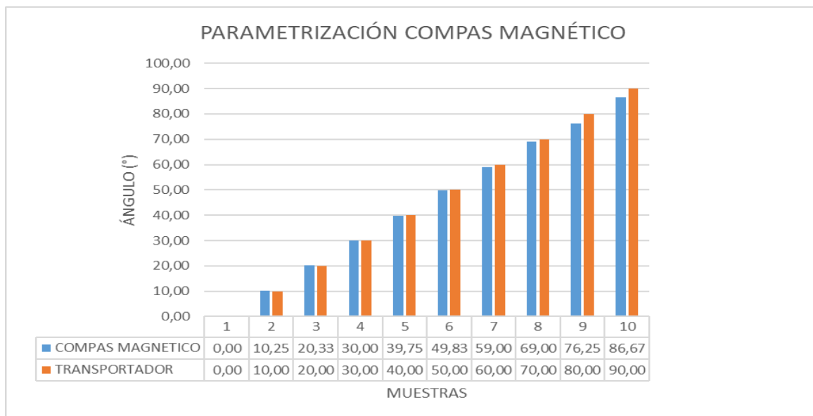
Figura 4. Obtención del error para el sensor compas magnético. (fuente de elaboración propia)
