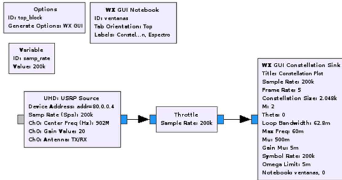
Figura 12. Diagrama de bloques recepción modulación constelaciones.
