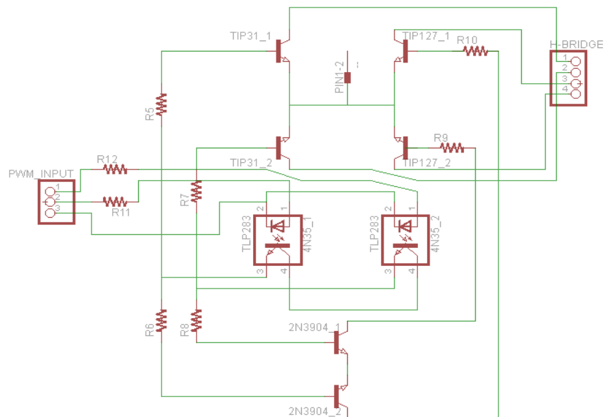
Figura 12 Esquema driver Puente H
