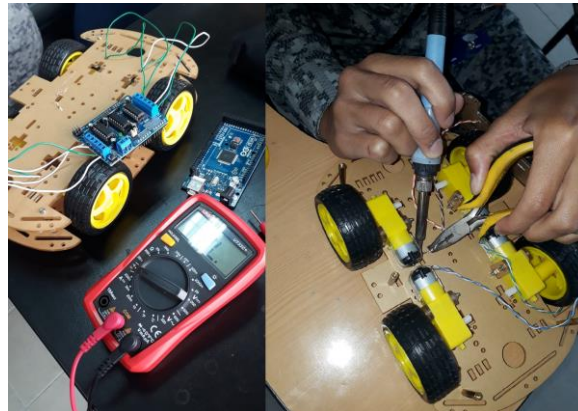
Figura 11. Ajustes y calibración del vehículo-robot. Fuente: elaboración propia de los autores.
