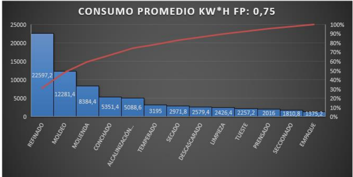
Figura 11. Potencia Promedio KW*h para un Factor de Potencia de 0,75
