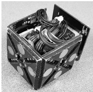
Fig. 1a. Modulo.
