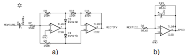
Figura 7. a) Etapa de rectificado y b) filtrado de la señal. Fuente: Brian Kaminski ARA/SED, 2014, “Muscle sensor V3”, Recuperado de: http://www.advancertechologies.com/p/muscle-sensor-v3.html
