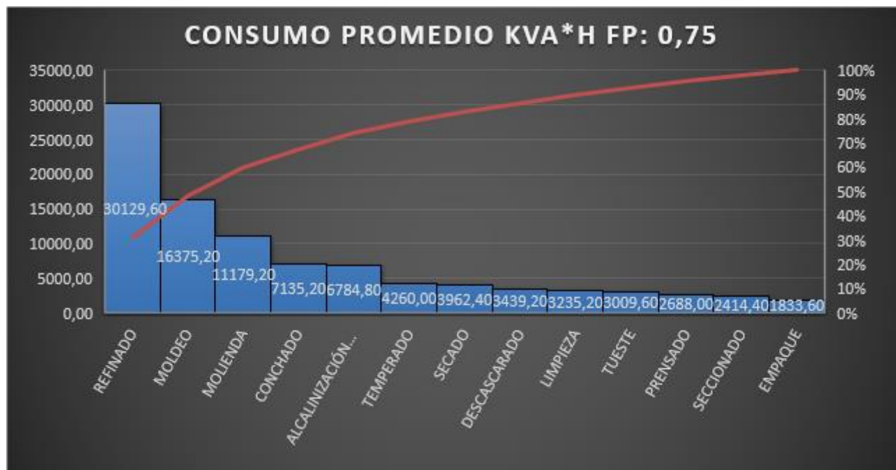
Figura 12. Potencia Promedio KVA*h para un Factor de Potencia de 0,75
