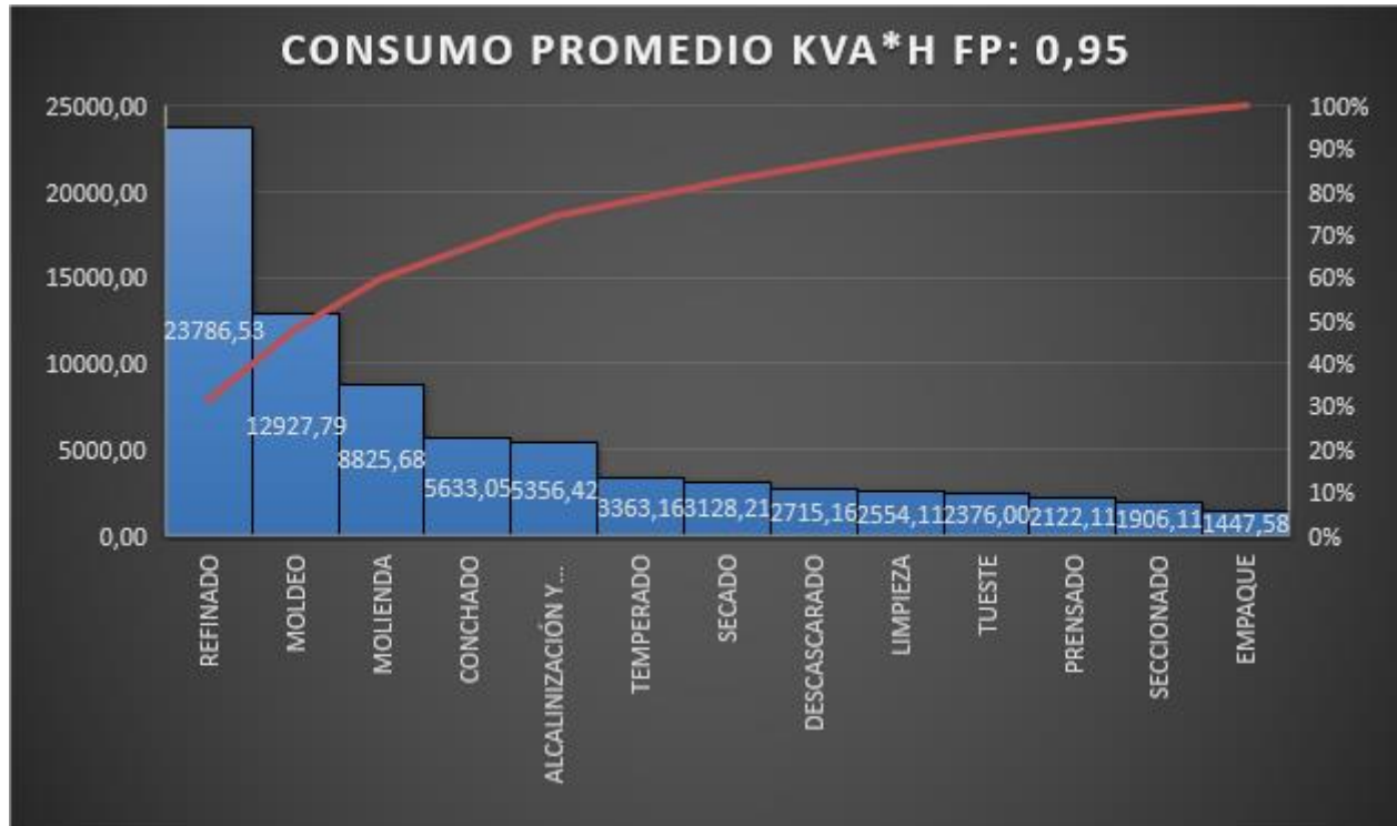
Figura 9. Potencia Promedio KVA*h para un Factor de Potencia de 0,95
