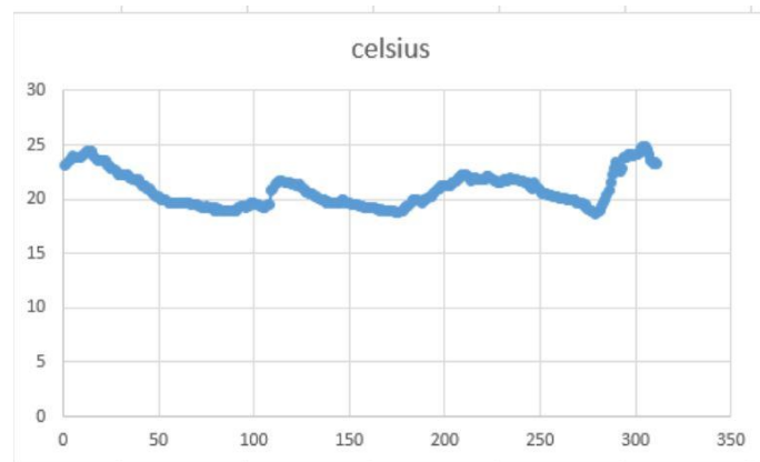
Figura 15. Comportamiento de la temperature. Fuente: Elaboración propia
