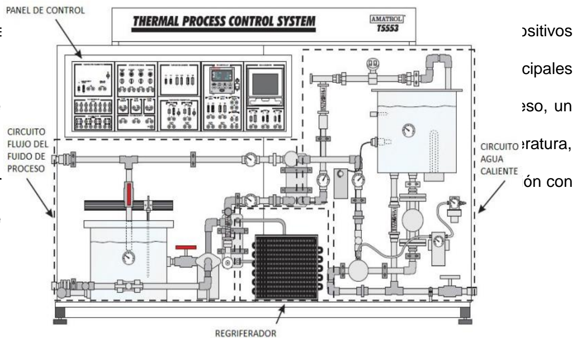
Figura 2. Planta Térmica como caso de estudio [21].
