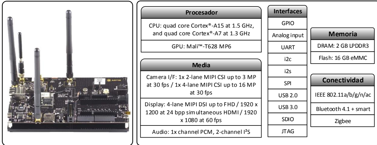
Figura 3. Principales especificaciones técnicas de la tarjeta Artik 1020
