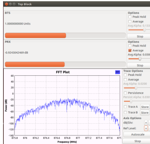
Figura 8. PUE dinámico malicioso
