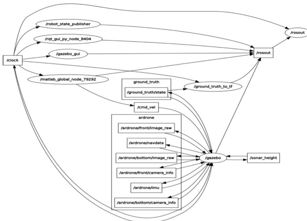
Figura 7. Nodos y Tópicos Correspondientes a la Integración Matlab-Gazebo. Autores
