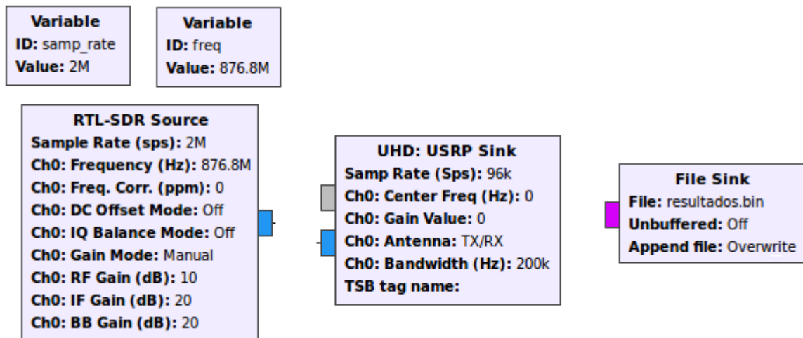
Figura 4. Componentes principales GNU Radio
