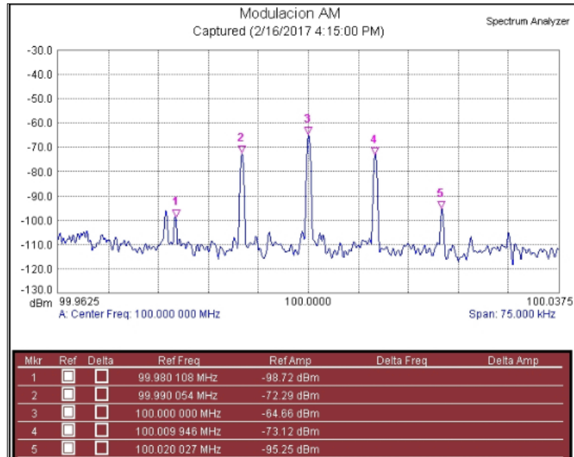
Figura 4. Modulación en amplitud AM
