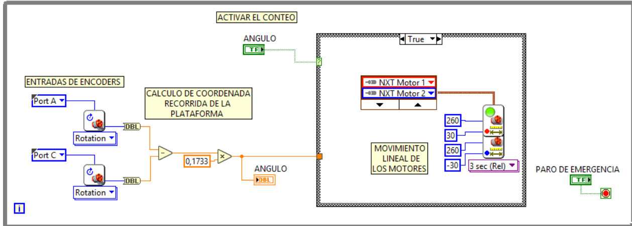
Figura 9. Algoritmo de ángulo recorrido por la plataforma maestro, implementado en LabVIEW®. [9]
