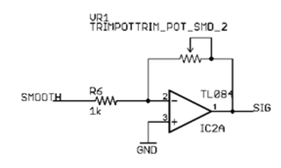
Figura 7. Circuito de ganancia de la señal. Fuente: Brian Kaminski ARA/SED, 2014, "Muscle sensor V3", Recuperado de: http://www.advancertechnologies.com/p/muscle-sensor-v3.html
