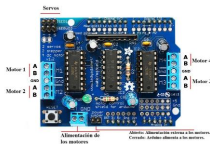
Figura 8. Se muestra el diagrama de pines de la tarjeta Shield. Fuente: Robots Didácticos, “Manejo de potencia para motores con el integrado L293D”, 2018, Recuperado de: http://robots-argentina.com.ar/didactica/manejo-de-potencia-para-motores-con-el-integrado-l293d/
