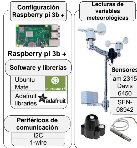
Figura 5. Principales características de los nodos inalámbricos
