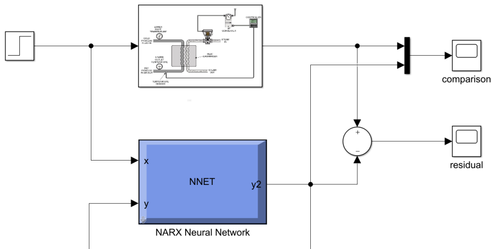
Figura 9. Esquema para detección de fallas en el accionamiento. Fuente: elaboración propia.
