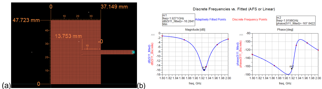
Figura 5. (a) Dimensiones de la antena (b) Resultado de la simulación. Fuente: Autor(es)
