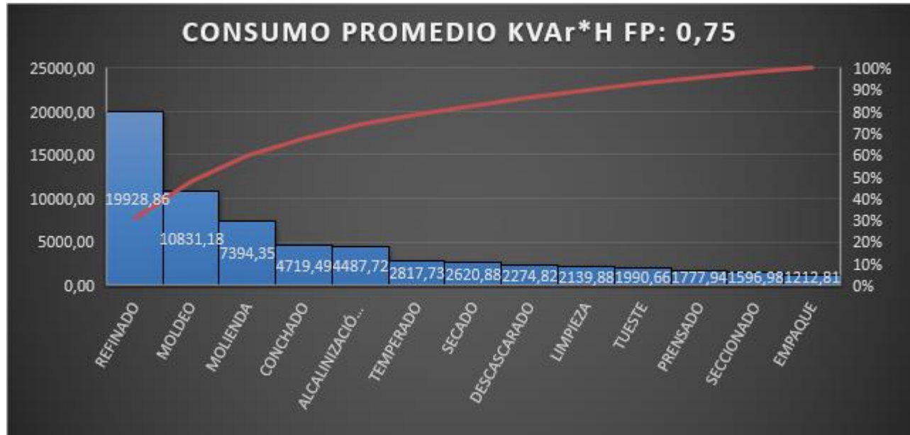
Figura 35. Potencia Promedio KVar*h para un Factor de Potencia de 0,75
