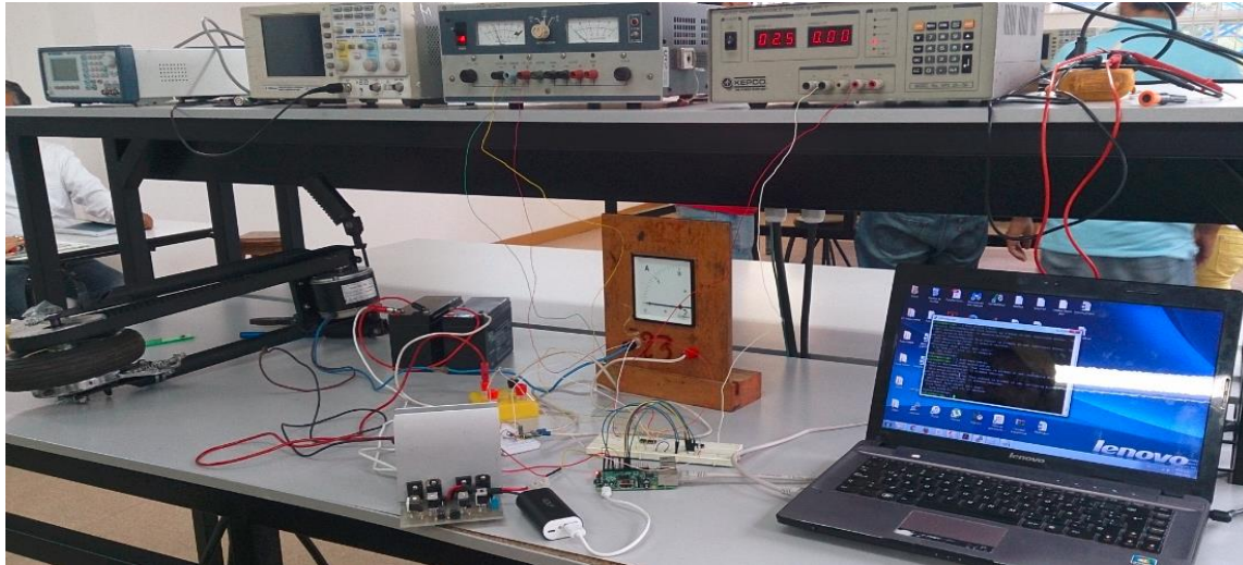
Figura 18 Implementación del prototipo de control de velocidad y torque a un motor DC
