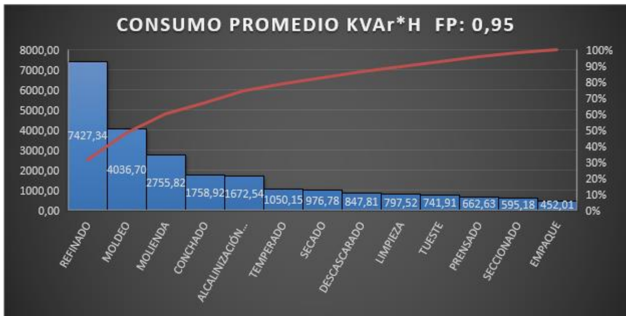
Figura 10. Potencia Promedio KVAR*h para un Factor de Potencia de 0,95
