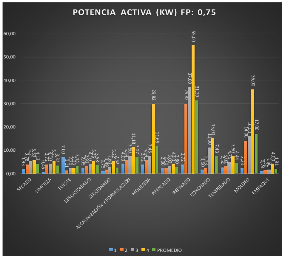
Figura 3. Potencia Activa para un Factor de Potencia de 0,75
