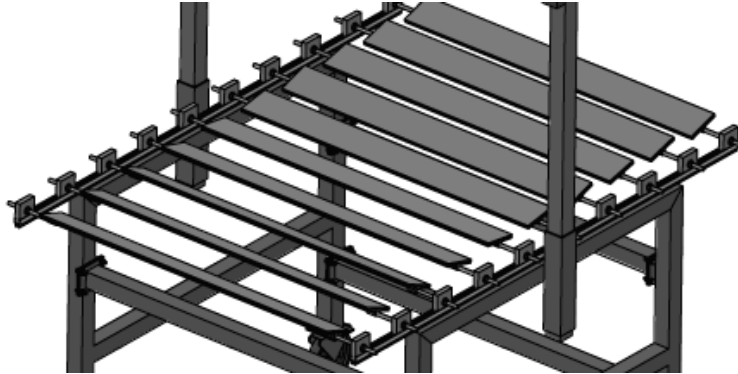
Figura 5 Modelado en CAD del sistema reflexión primario. Fuente: elaborado por los autores
