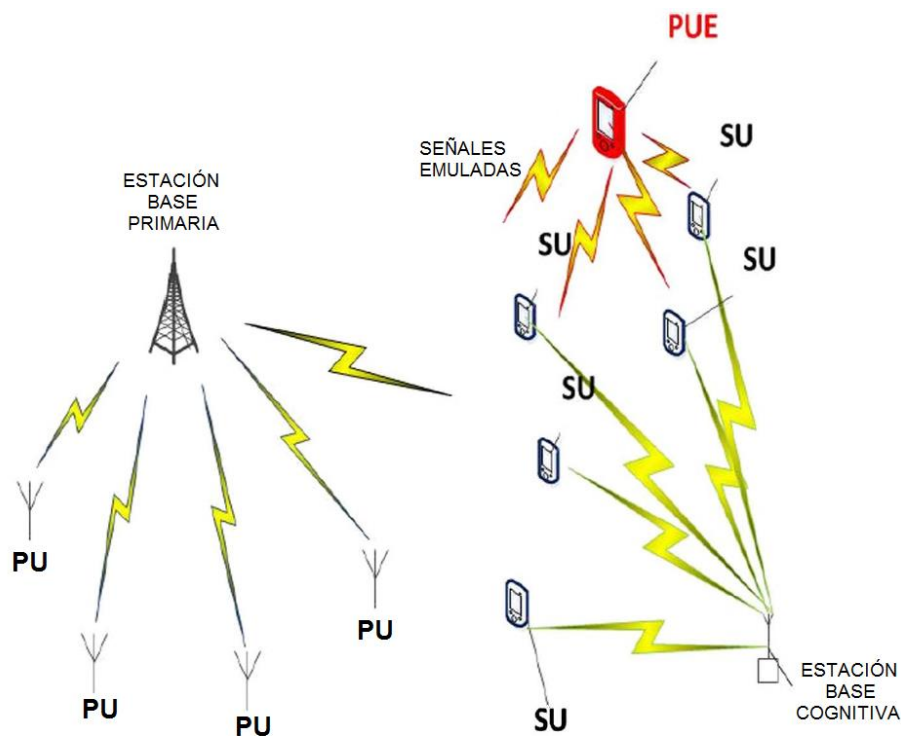
Figura 2. Estructura general del ataque de emulación de usuario primario [14].
