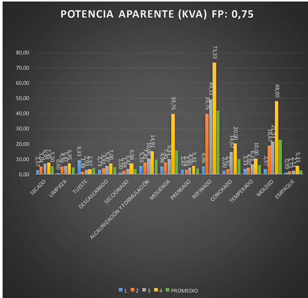
Figura 5. Potencia Aparente para un Factor de Potencia de 0,75
