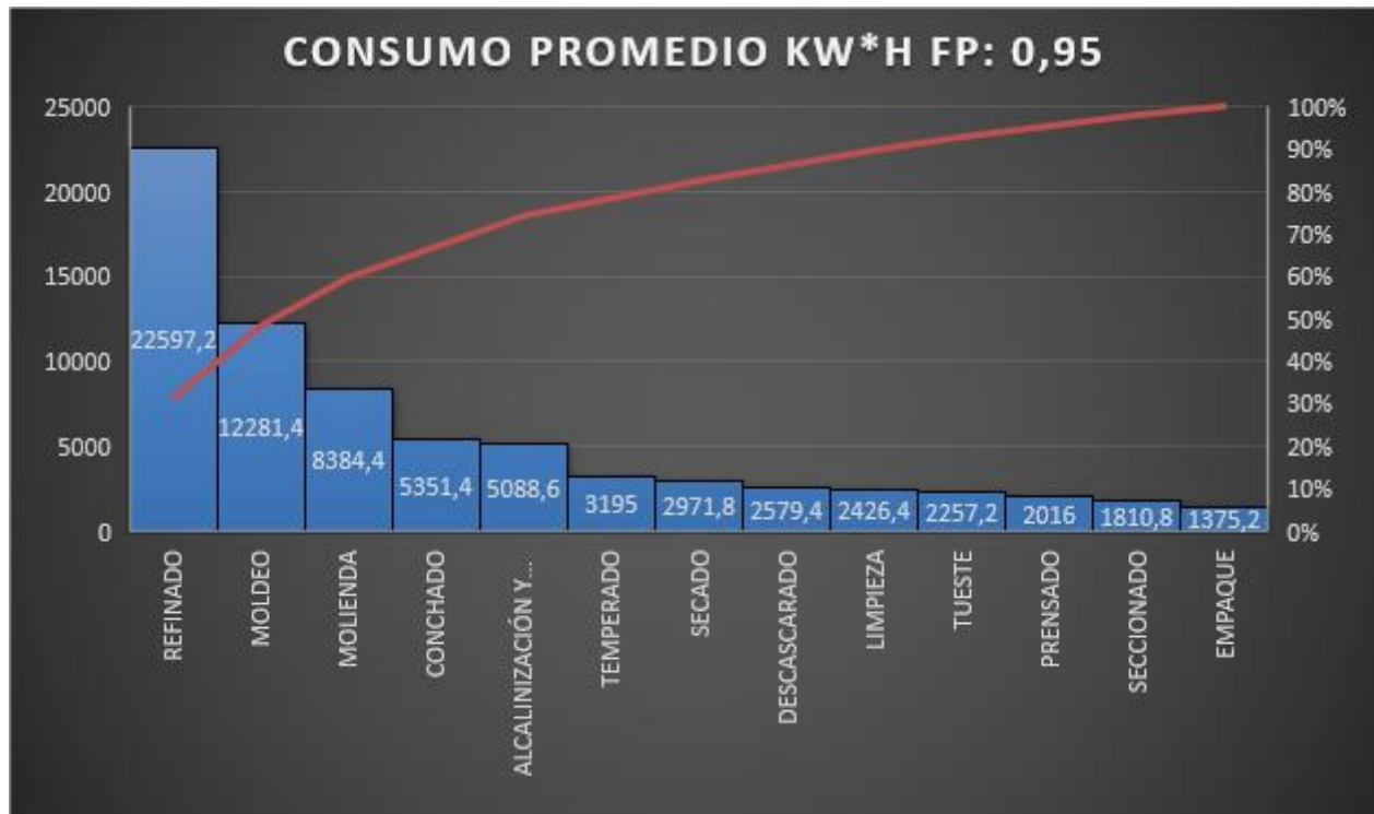
Figura 8. Potencia Promedio Kw*h para un Factor de Potencia de 0,95
