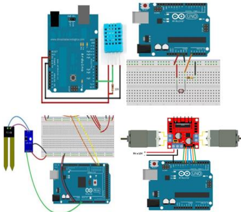
Figura 11. DHT11, LDR, Humedad del suelo, puente H. Fuente: [4]
