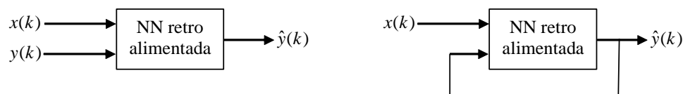
(a) Arquitectura serie-paralelo
