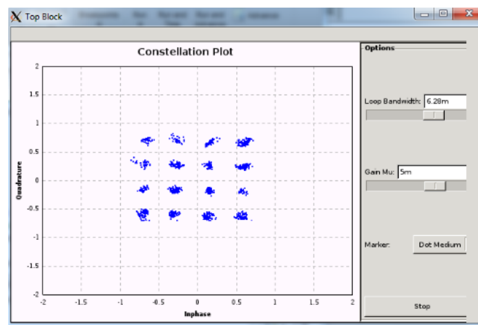
Figura 15.3 Constelación modulación 16QAM
