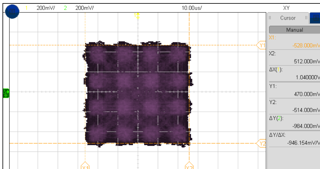
Figura 10. Modulación 16QAM.
