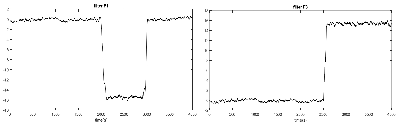
Figura 12. Evaluación de fallas F1 y F3. Fuente: elaboración propia.
