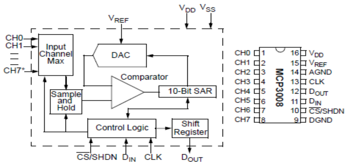
Figura 16 Esquema convertidor de señal analógico digital
