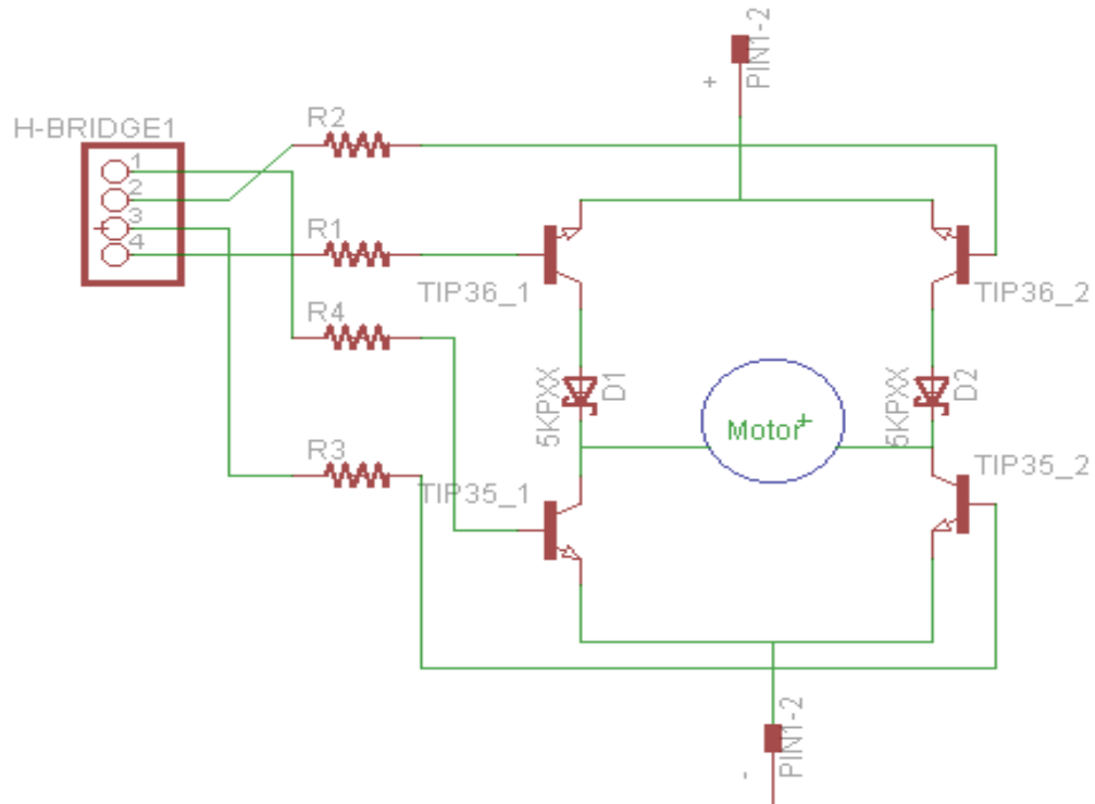
Figura 13 Esquema Puento H
