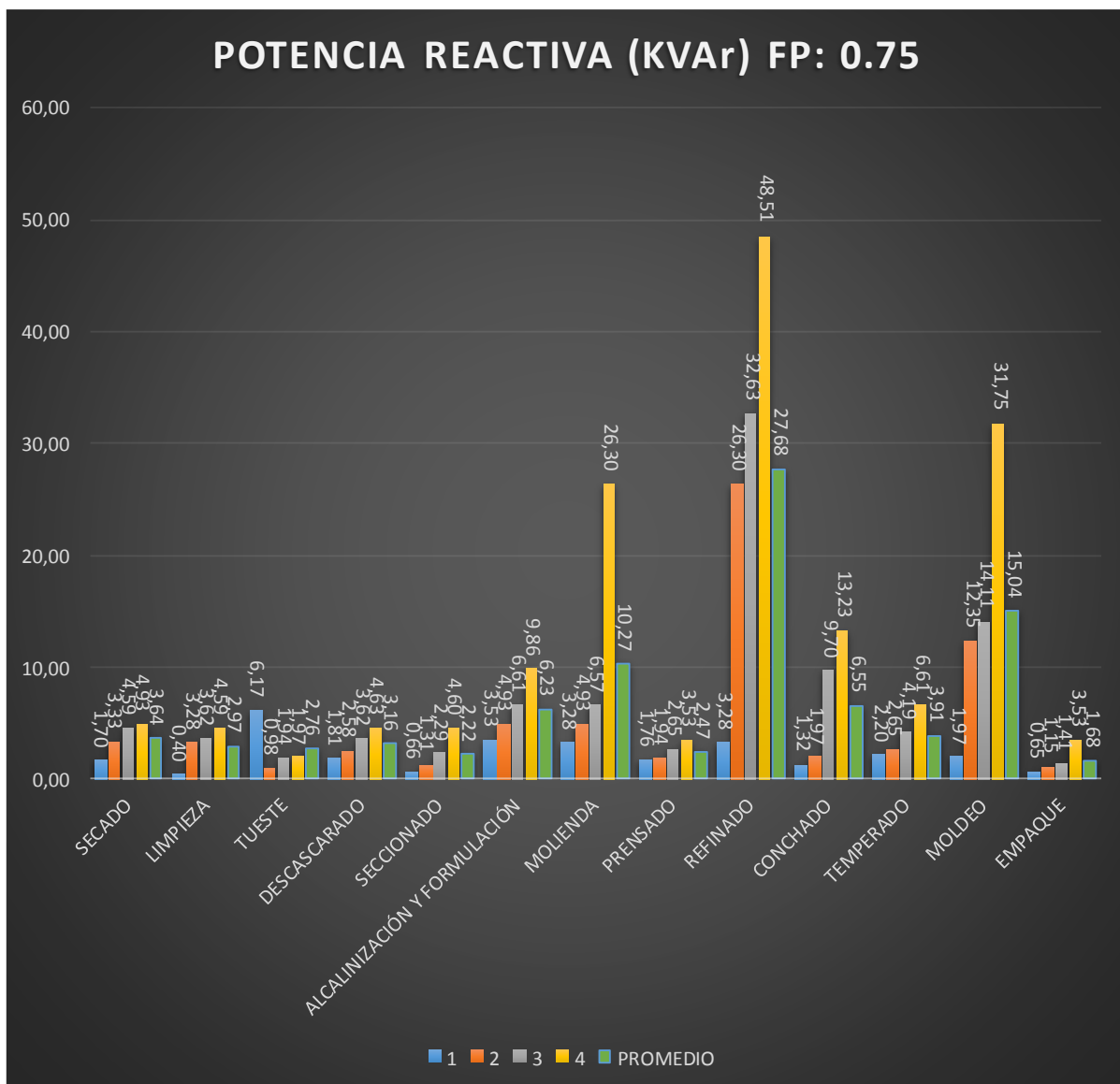
Figura 7. Potencia Reactiva para un Factor de Potencia de 0,75
