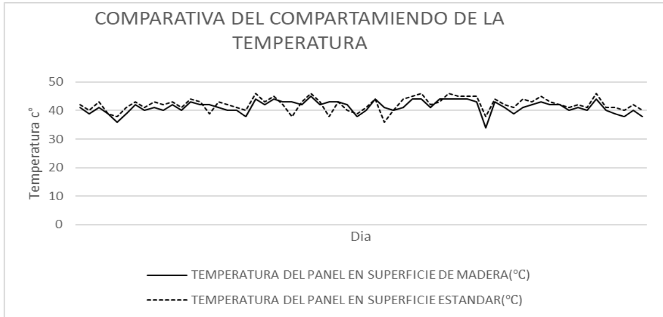
Gráfico 5 Comparativa de la temperatura generada. (Datos recolectados 5:00 pm) Fuente: elaboración propia de los autores.
