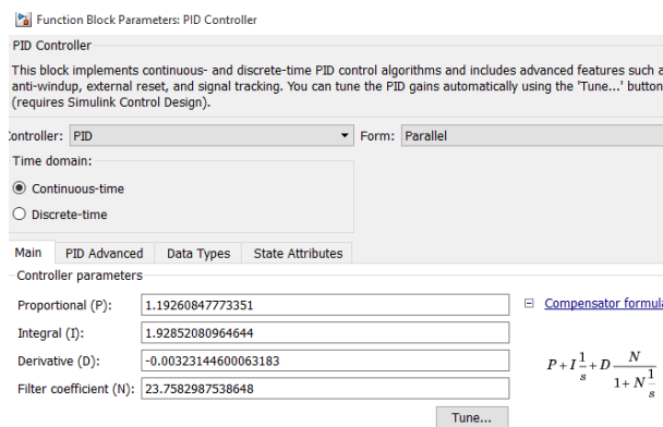
Figura 2 Sintonización automática de constantes SIMULINK/MATLAB
