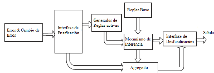
Figura 4 Controlador Difuso
