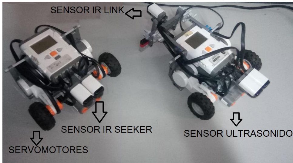
Figura 2. Robots esclavos. (fuente de elaboración propia)
