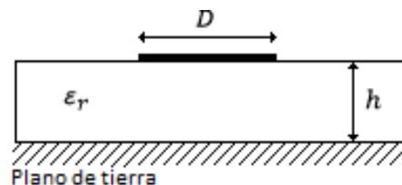
Figura 2. Dimensiones líneas microstrip. Fuente: Autor(es)[24]
