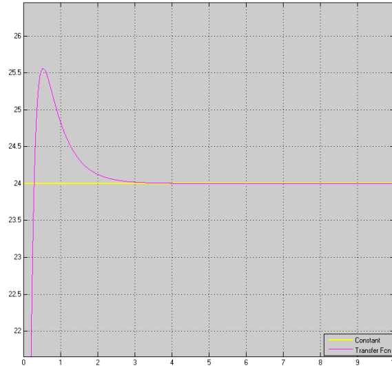
Figura 3 Respuesta de la planta controlada y señal de referencia en SIMULINK/MATLAB
