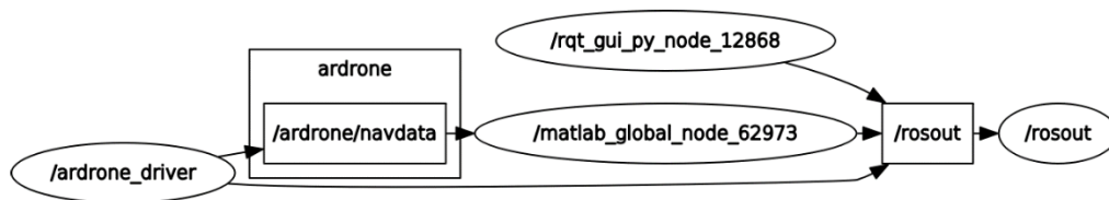
Figura 6. Nodo Matlab para el control del ArDrone. Autores
