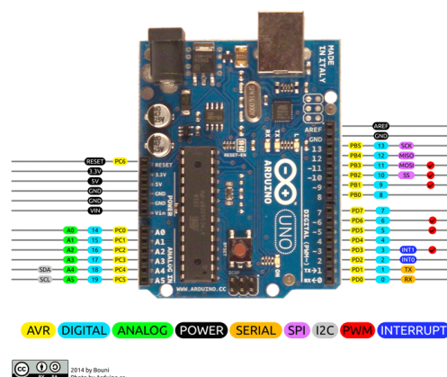
Figura 8. Se muestra el diagrama de pines del Arduino uno. Fuente: Components101, "Arduino Uno", 2018, Recuperado de: https://components101.com/microcontrollers/arduino-uno .
