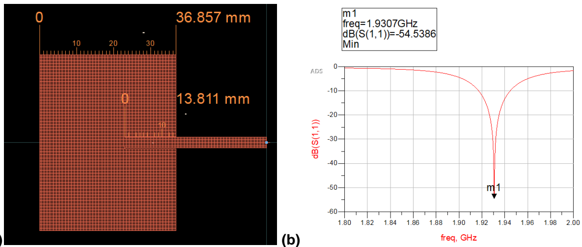
Figura 14. (a) Dimensiones finales de la antena (b) Sintonización de S_{11} variando L. Fuente: ADS Software
