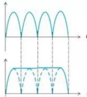
Figura 6. Nos indica la señal de entrada en el circuito del filtro paso bajo y la señal a la salida del circuito paso bajo. Fuente: emgprotesisdmm, “¿cómo hacer su propio circuito sensor de músculo / EMG?”, 2016, Recuperado de: https://emgprotesisdmm.wordpress.com/2016/08/02/como-hacer-su-propio-circuito-sensor-de-musculo-emg/ .
