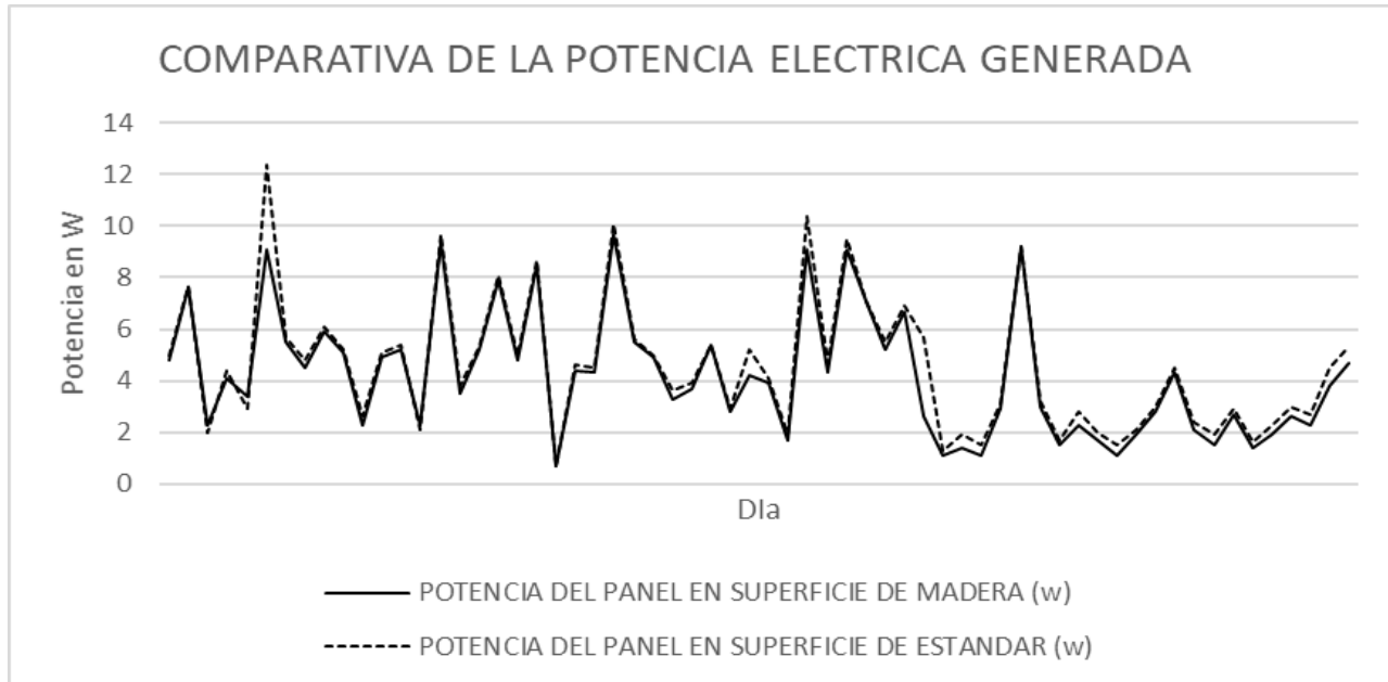
Gráfico 6 Comparativa de la potencia eléctrica generada. (Datos recolectados 12:00 m)
