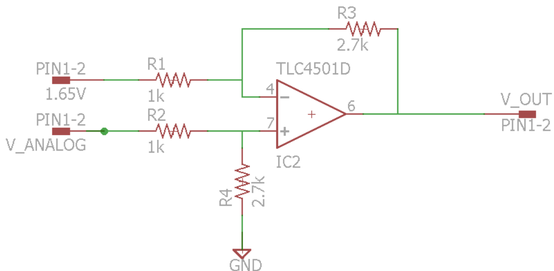
Figura 17 Circuito acondicionador de señal
