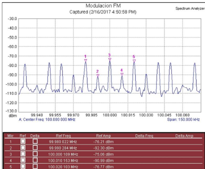
Figura 5. Modulación en frecuencia FM
