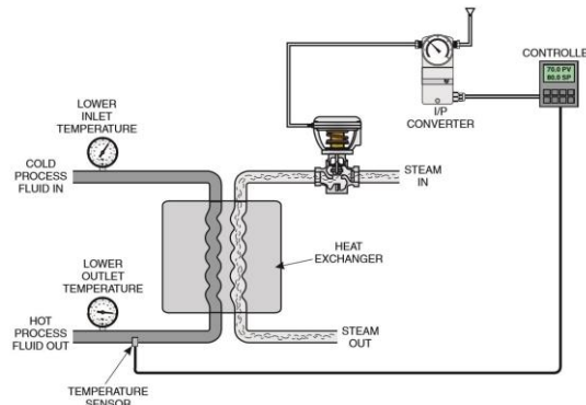
Figura 3. Sistema de control de temperatura del proceso térmico [21].
