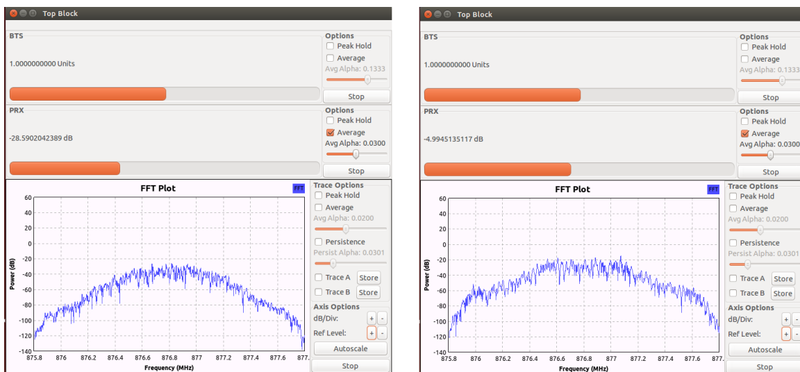
Figura 6. MCRN sin PUE y con PUE malicioso
