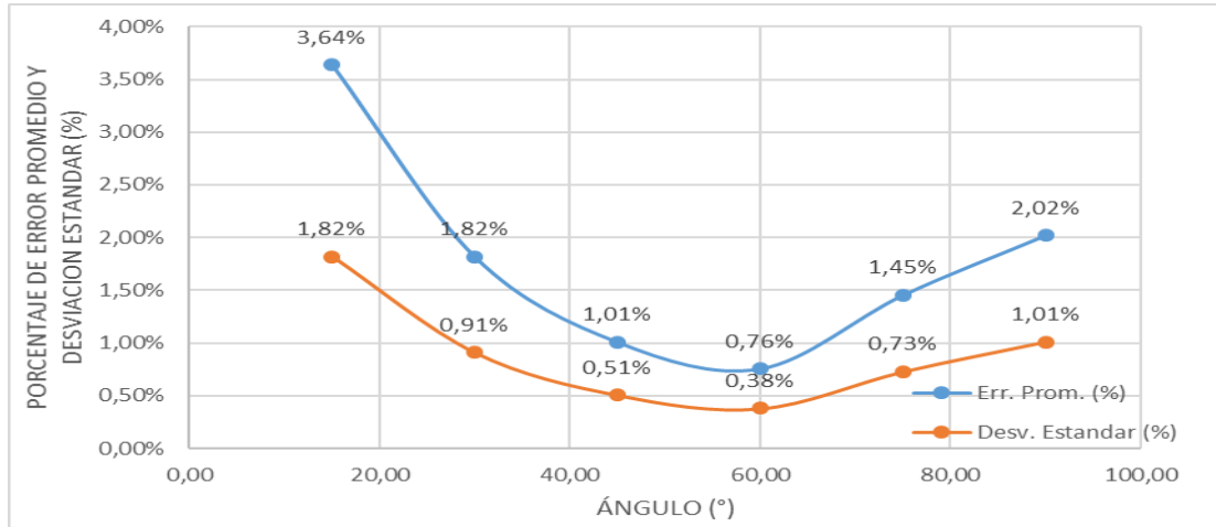
Figura 11. Error promedio y desviación estándar del movimiento angular
