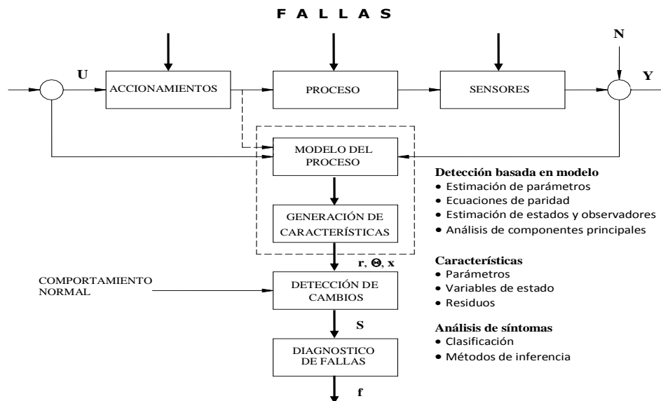
Figura 1. Esquema general de un sistema de detección and diagnóstico de fallas. Fuente: elaboración propia.
