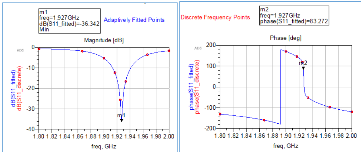
Figura 11. Simulación inicial de la segunda antena. Fuente: ADS Software
