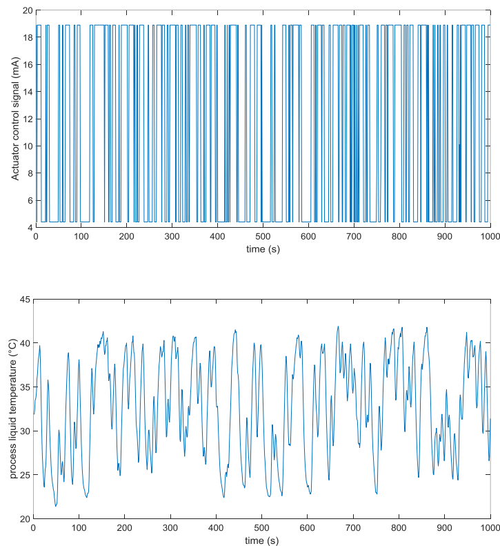
Figura 6. Datos de entrada/salida durante la operación del equipo. Fuente: elaboración propia.
