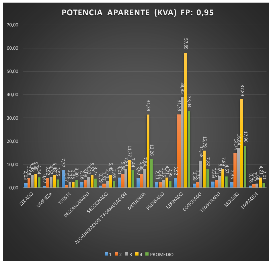
Figura 4. Potencia Aparente para un Factor de Potencia de 0,95
