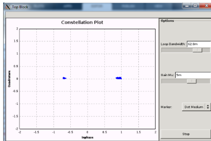
Figura 14. Constelación modulación BPSK.
