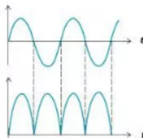
Figura 5. Nos indica la señal de entrada en al circuito rectificador y la señal a la salida del circuito rectificador. Fuente: emgprotesisdmm, "¿cómo hacer su propio circuito sensor de músculo / EMG?", 2016, Recuperado de: https://emgprotesisdmm.wordpress.com/2016/08/02/como-hacer-su-propio-circuito-sensor-de-musculo-emg/
