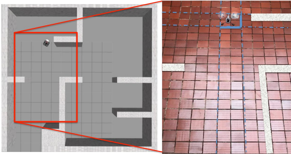
Figura 11. Simulación Gazebo y parte del escenario real para la Ruta 3. Autores
