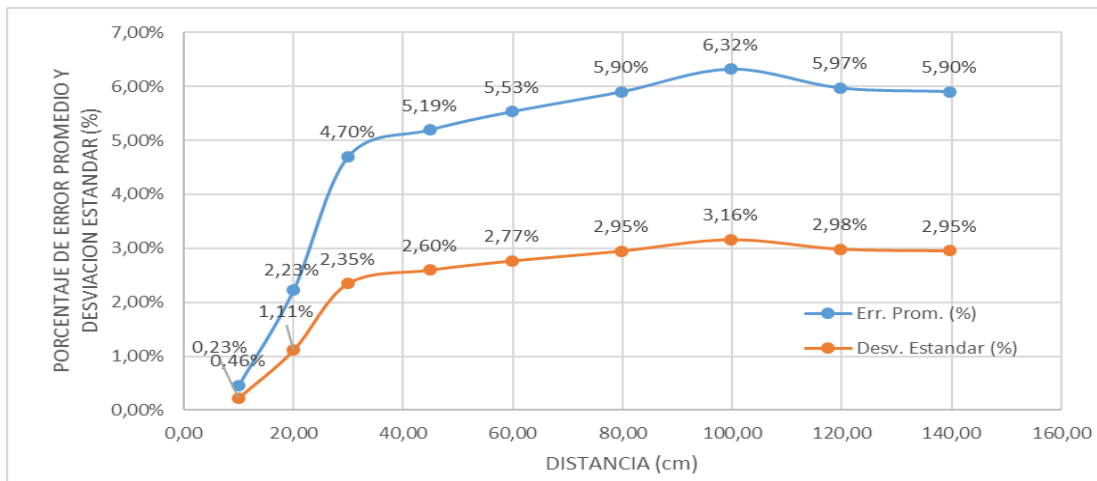
Figura 10. Error promedio y desviación estándar del movimiento lineal
