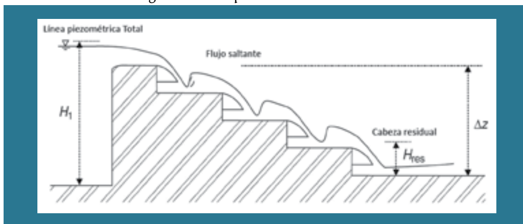
Figura B. 6.4 Esquema de caída escalonada 3
