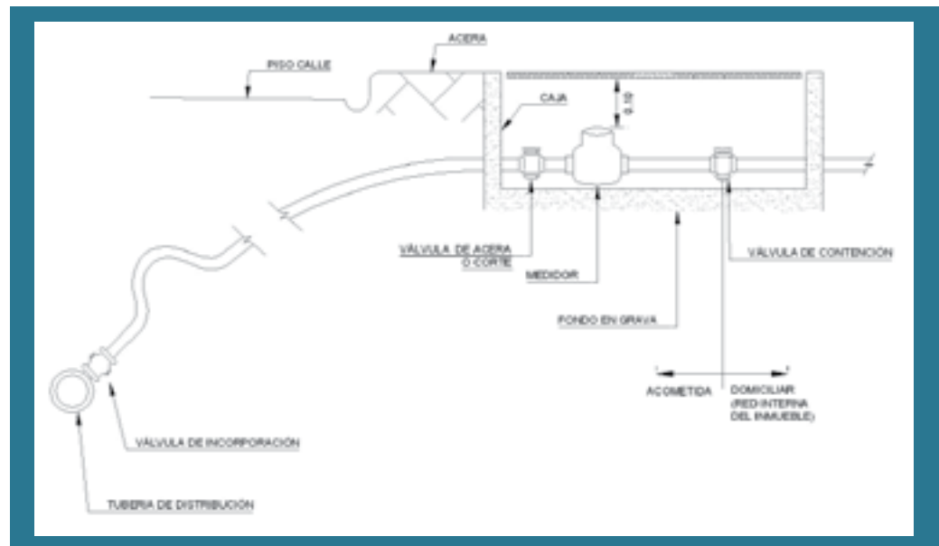
Figura B. 7.4 Esquema de Acometida Diámetro 13 mm.
