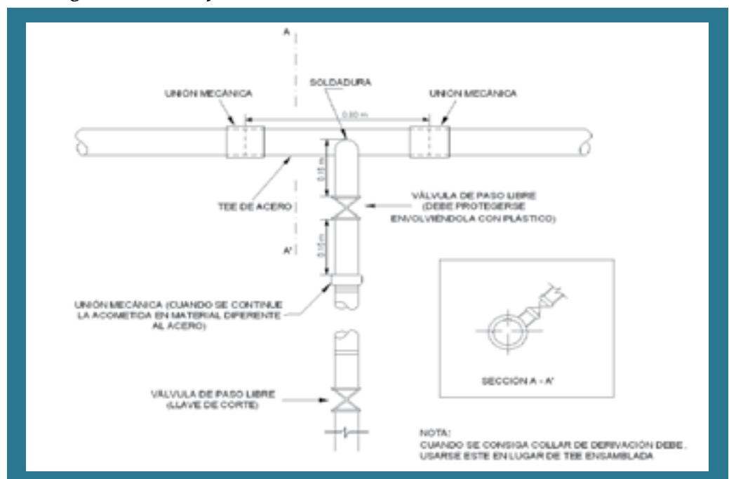
Figura B. 7.5 Esquema de Acometida utilizando derivación en TEE
