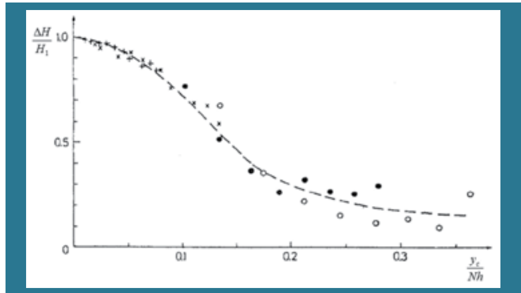
Figura B. 6.5 Relación entre porcentaje de disipación y altura caída 5
