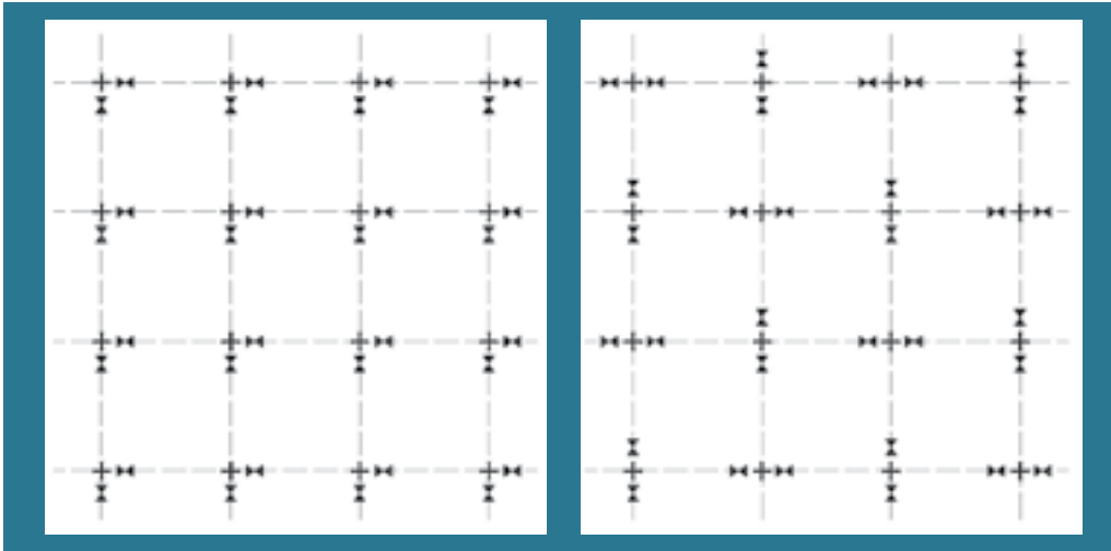
Figura B. 7.1 Disposición de válvulas para redes de distribución de 75 y 100 mm de diámetro
