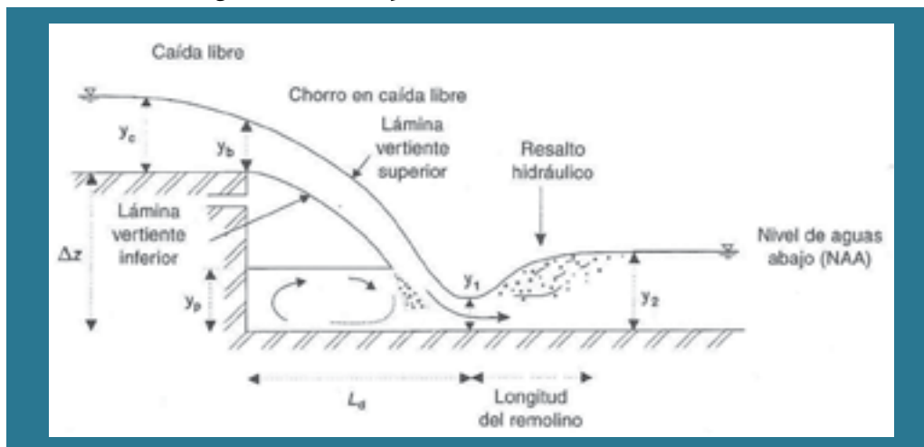
Figura B. 6.3 Esquema de estructura de caída 3
