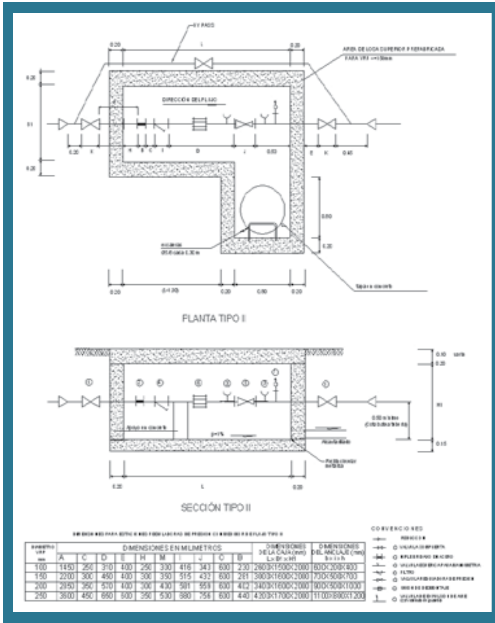
Figura B. 7.3 Esquema Estación Reguladora de Presión para d = 100, 150, 200 y 250 mm.
