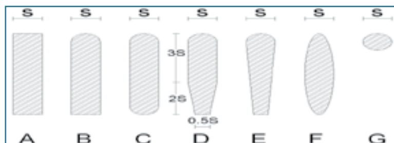
Figura B. 4.1 Diferentes formas de barros de rejillas
