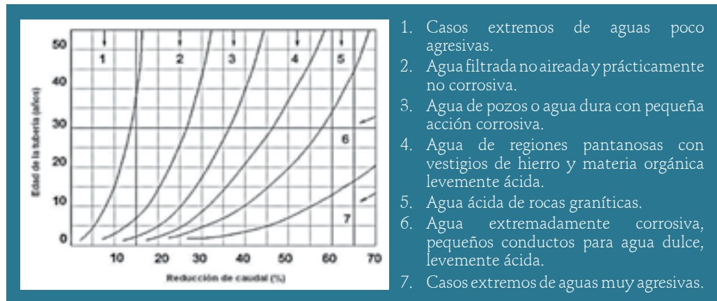
Figura B. 6.1 Reducción del caudal en función de la edad de la tubería
