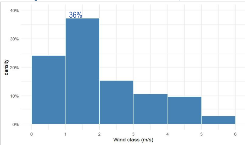
Figura 9. Distribución frecuencial de velocidad del viento, abril 2025.
