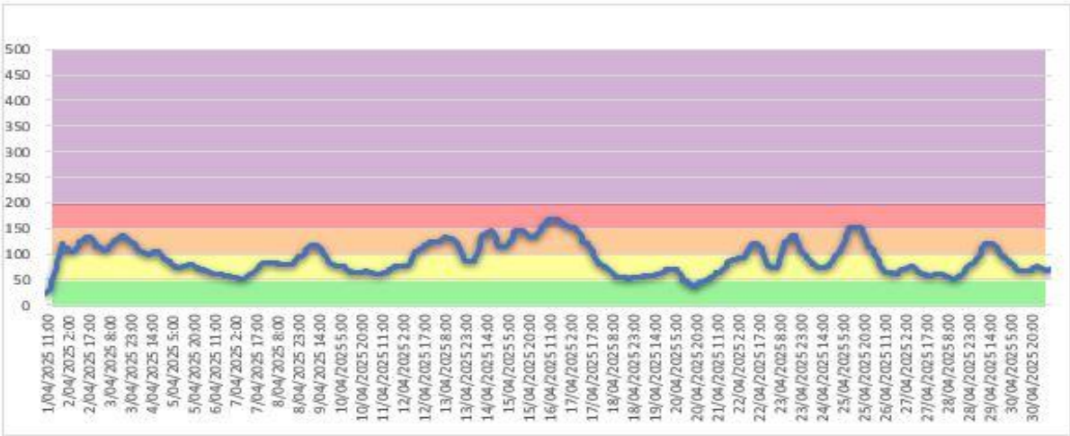
Figura 6. Índice de Calidad del Aire, determinado por el IBOCA pm_{10} . abril de 2025.
