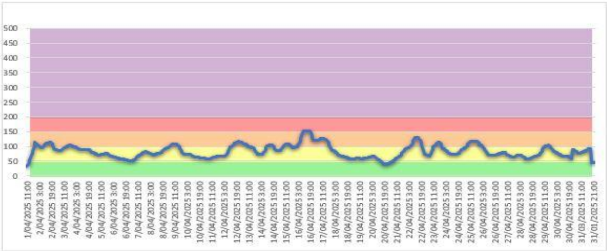
Figura 7. Índice de Calidad del Aire, determinado por el IBOCA pm_{10} . abril de 2025.
