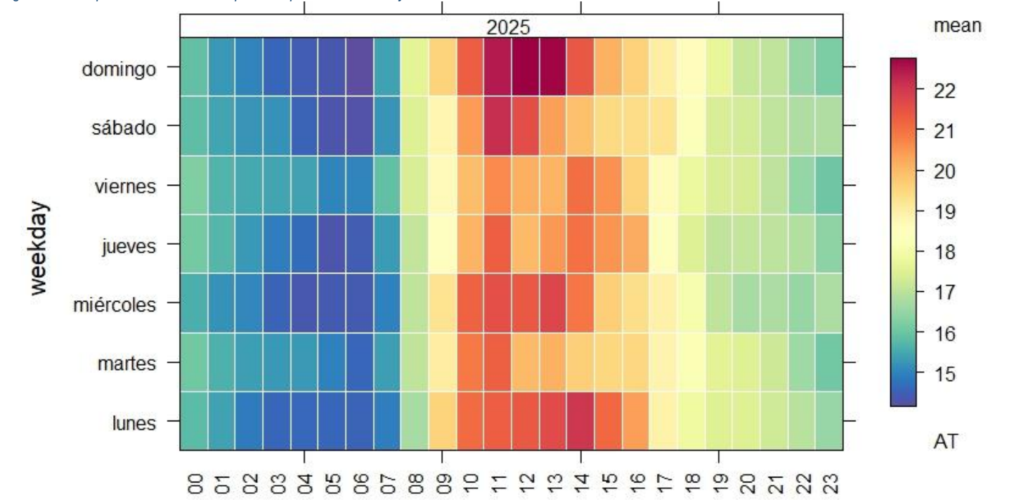
Figura 13. Comportamiento de la Temperatura promedio horario y semanal. abril 2025
