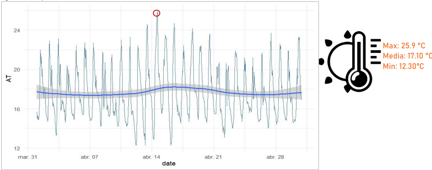
Figura 12. Temperatura Ambiente en °C. abril 2025.
