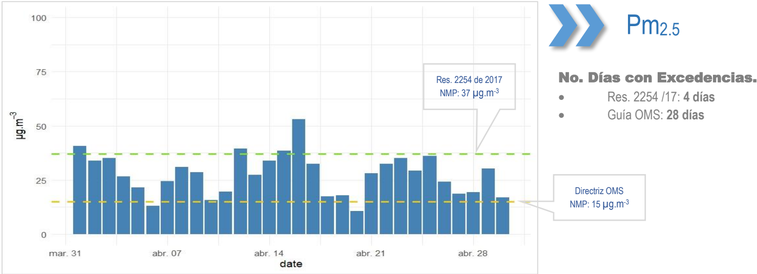
Figura 5. Nivel máximo permisible para pm_{2.5} . abril 2025.
