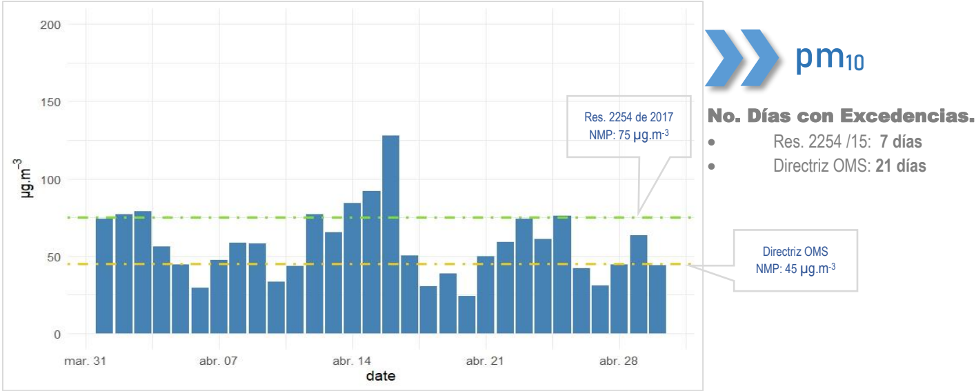
Figura 4. Nivel máximo permisible para pm_{10} . abril 2025.
