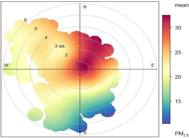
Figura 11. Diagrama polar pm2.5 en relación a la rosa de los vientos
