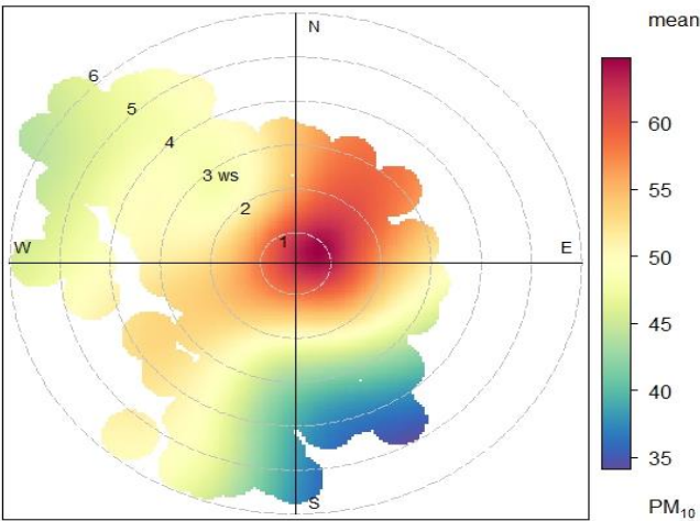
Figura 10. Diagrama polar pm10 en relación a la rosa de los vientos.
