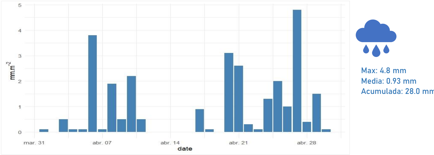
Figura 14. Precipitación acumulada 24 horas. abril 2025.
