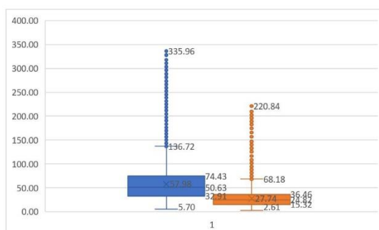
Figura 2. Boxplot pm_{10} y pm_{2.5} . abril 2025.
