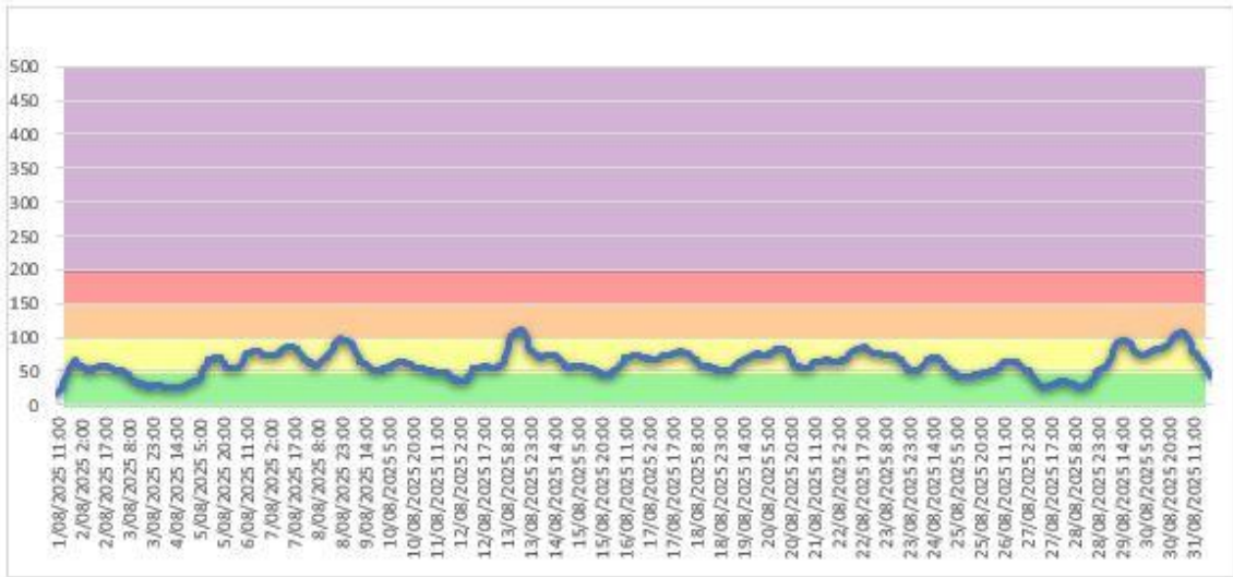
Figura 7. Índice de Calidad del Aire, determinado por el IBOCA pm_{10} . Agosto de 2025.
