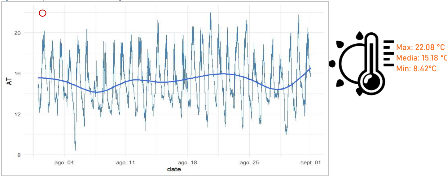
Figura 12. Temperatura Ambiente en °C. Agosto 2025.
