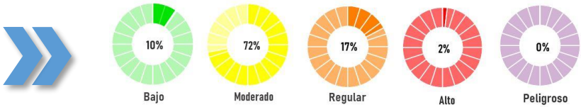
Figura 7. Índice de Calidad del Aire, determinado por el IBOCA pm_{10} . Agosto de 2025.
