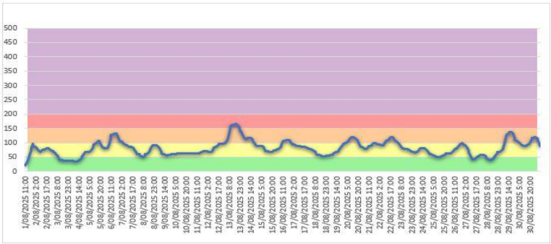
Figura 6. Índice de Calidad del Aire, determinado por el IBOCA pm_{10} . Agosto de 2025.
