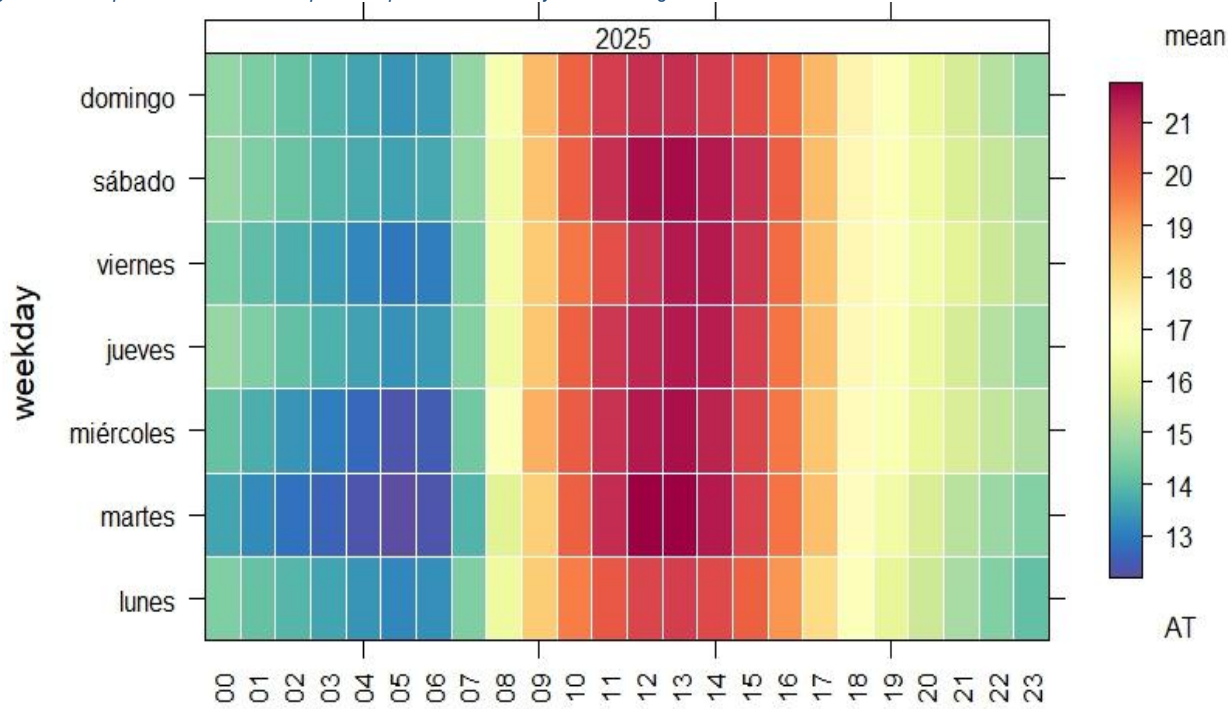
Figura 13. Comportamiento de la Temperatura promedio horario y semanal. Agosto 2025
