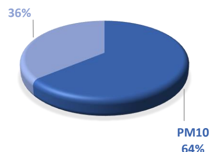
Figura 2. Fracción de material particulado
