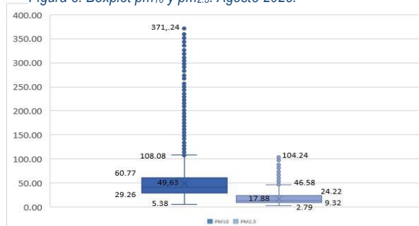
Figura 3. Boxplot pm_{10} y pm_{2.5} . Agosto 2025.
