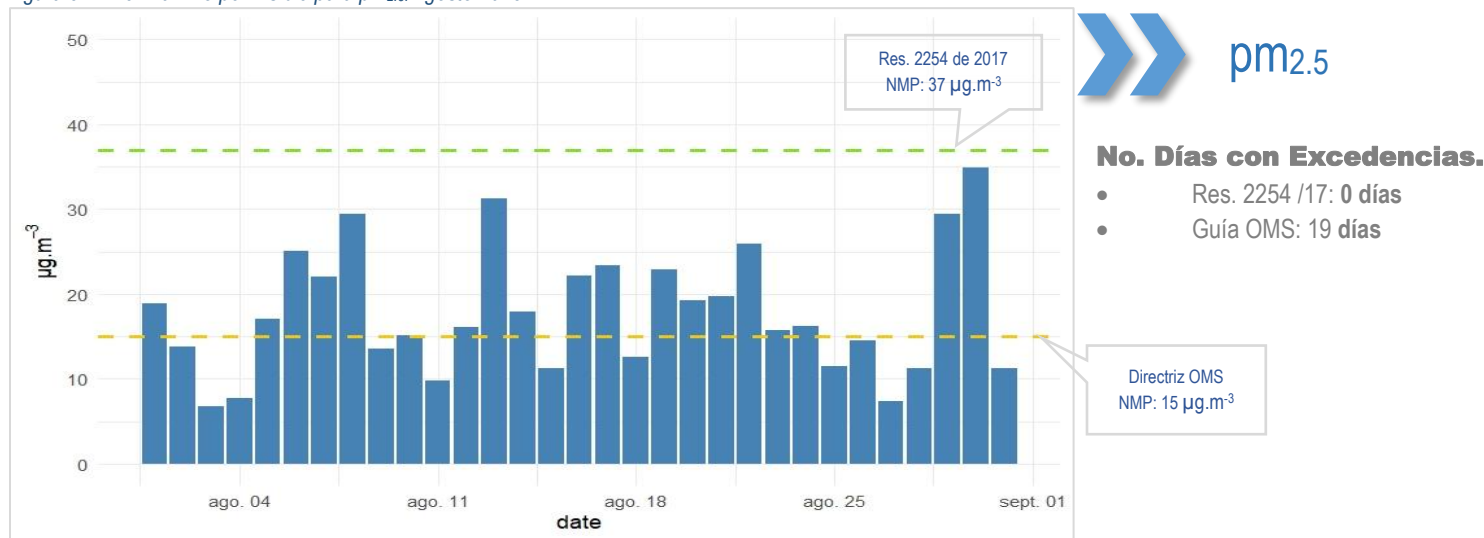
Figura 5. Nivel máximo permisible para pm_{2.5} . Agosto 2025.
