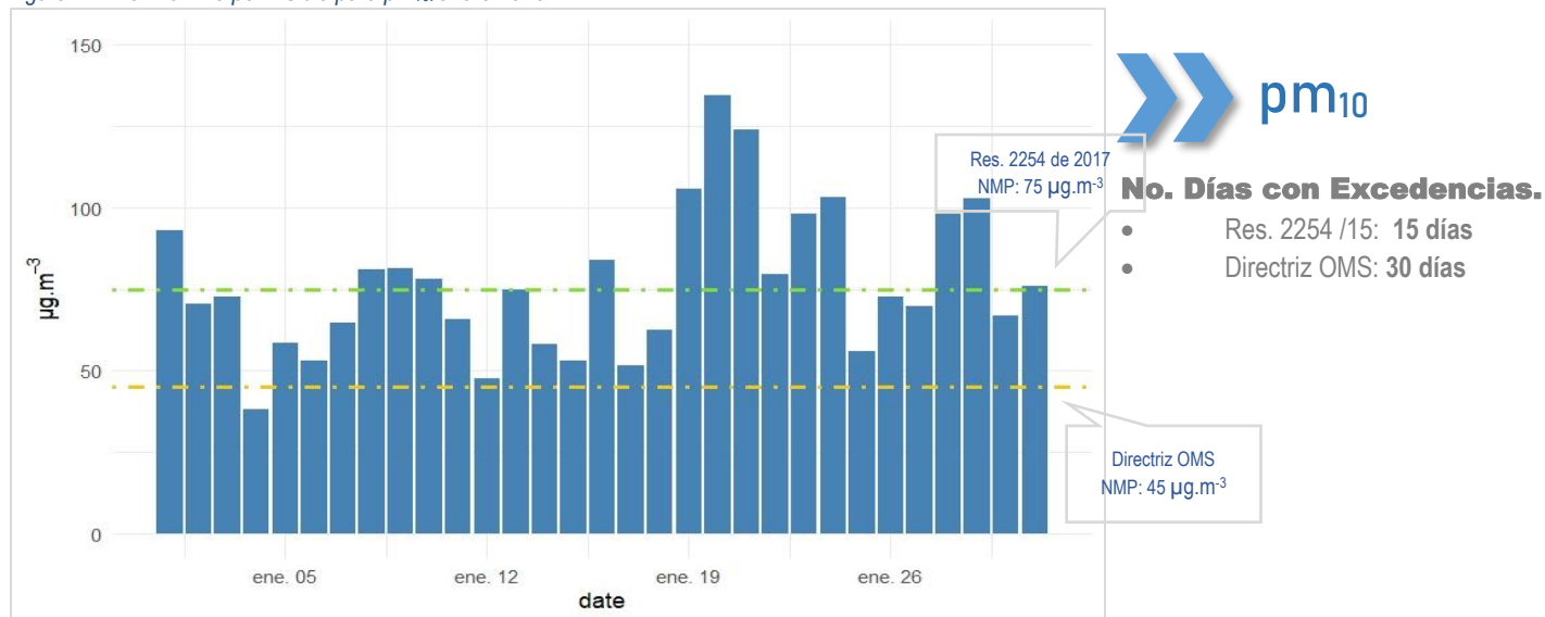
Figura 4. Nivel máximo permisible para pm_{10} enero 2026.
