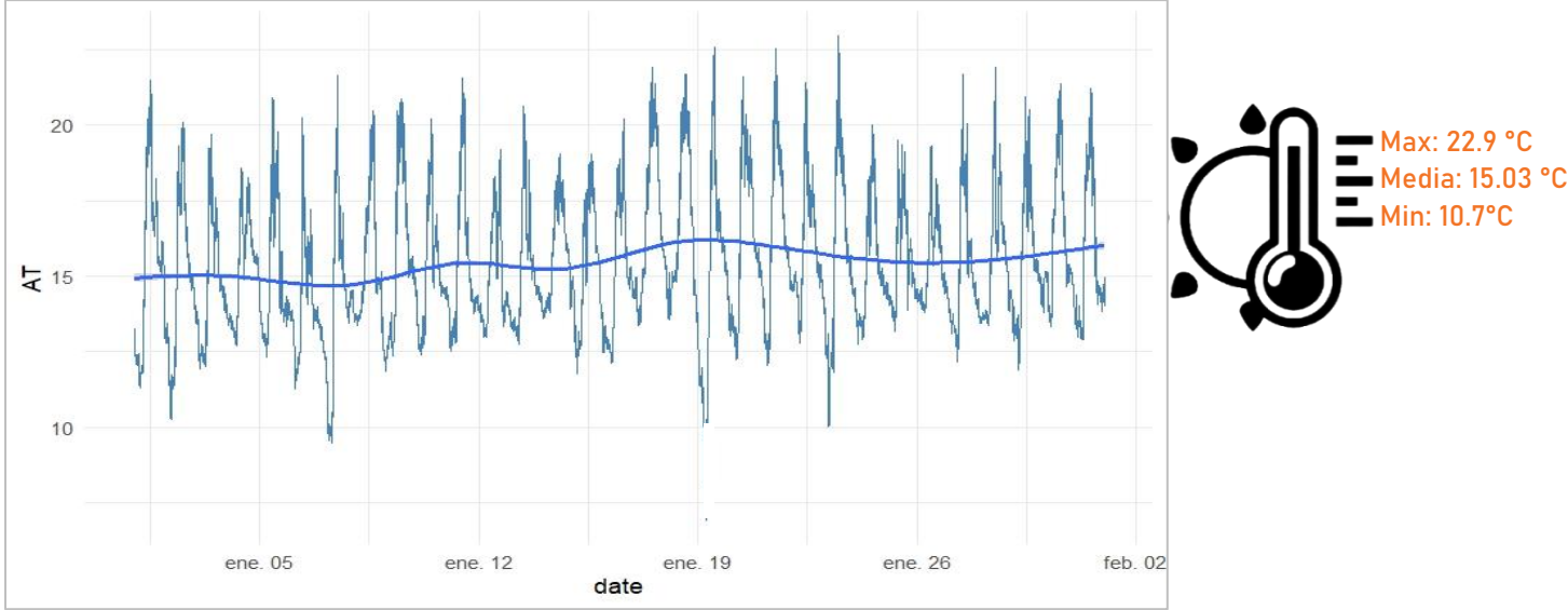
Figura 12. Temperatura Ambiente en °C. enero 2026.
