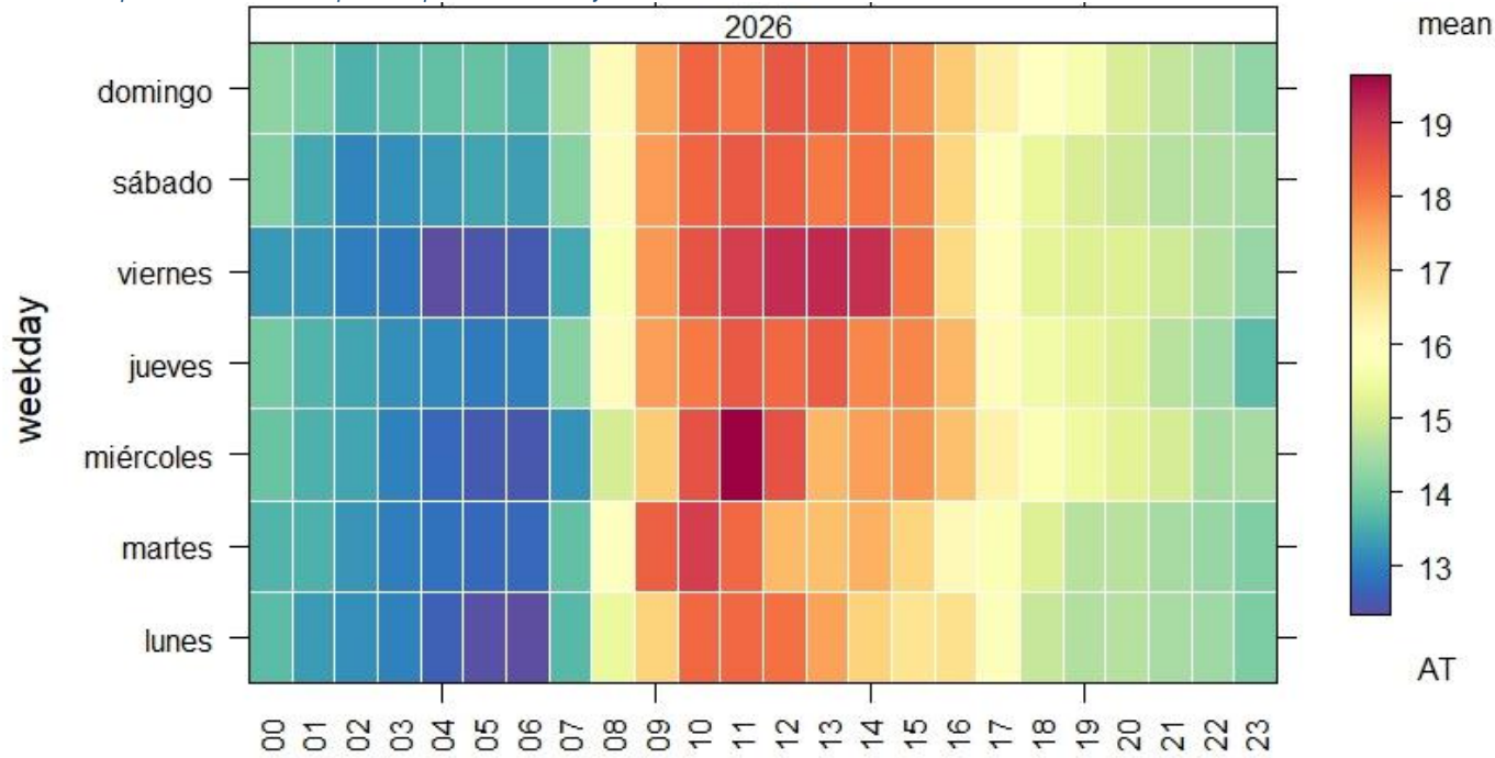
Figura 13. Comportamiento de la Temperatura promedio horario y semanal. enero 2026.
