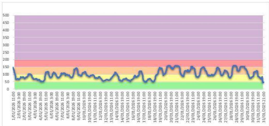
Figura 7. Índice de Calidad del Aire, determinado por el IBOCA pm_{10} . enero de 2026.
