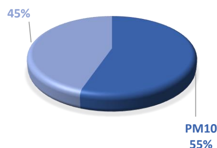
Figura 2. Fracción de material particulado
