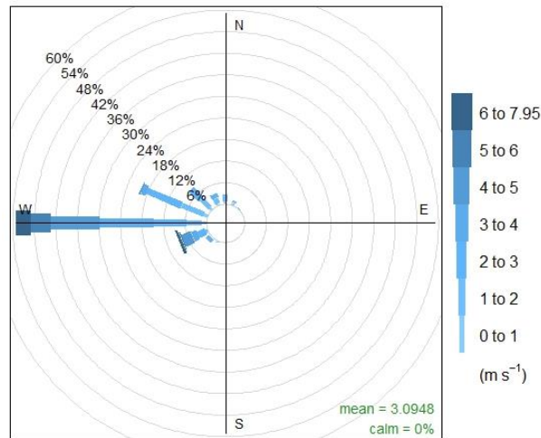
Figura 8. Rosa de los vientos, enero 2026.
