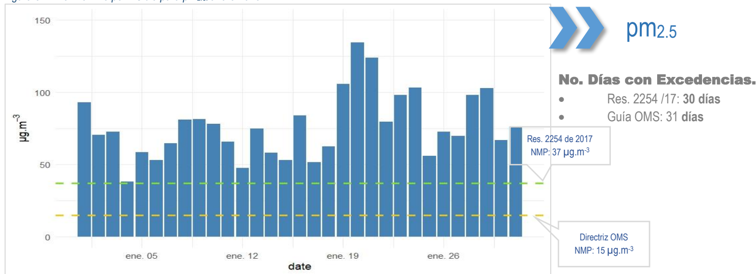
Figura 5. Nivel máximo permisible para pm_{2.5} enero 2026.
