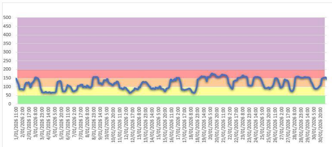
Figura 6. Índice de Calidad del Aire, determinado por el IBOCA pm_{10} . enero de 2026.
