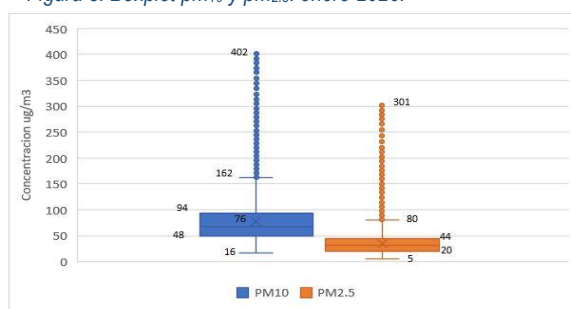
Figura 3. Boxplot pm_{10} y pm_{2.5} . enero 2026.
