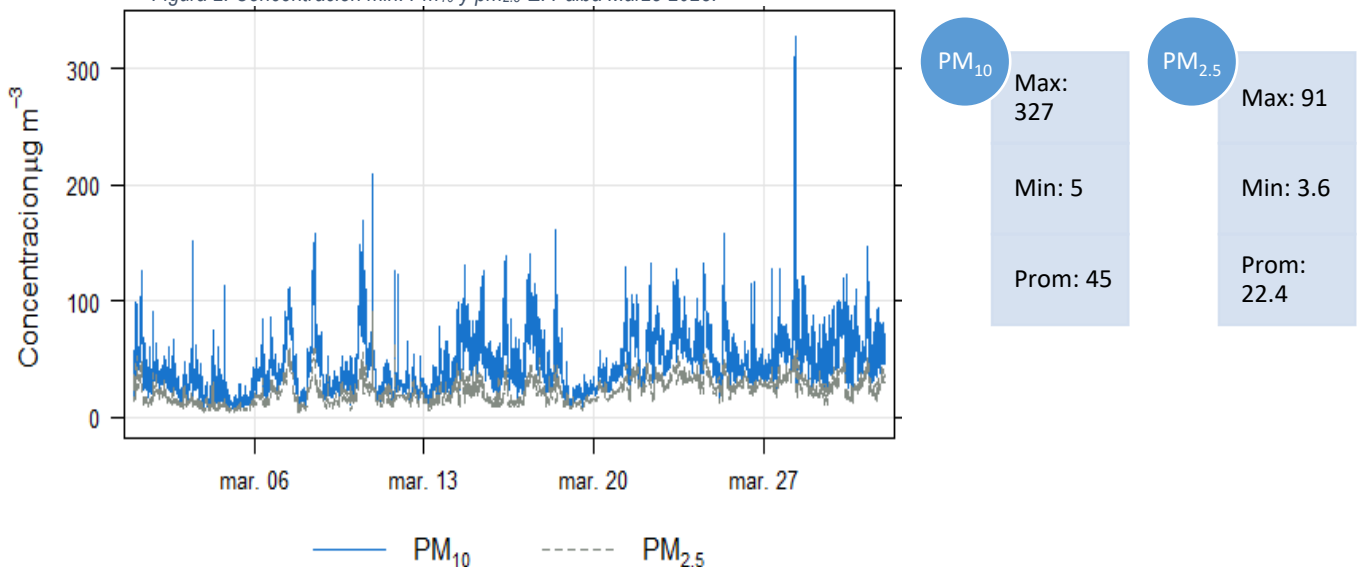
Figura 2: Concentración min. Pm 10 y pm 2.5 E. Paiba Marzo 2023.
