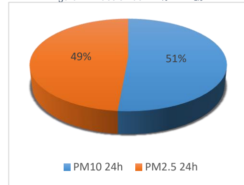
Figura 4: Fracción de PM 10 Y PM 2.5 .
