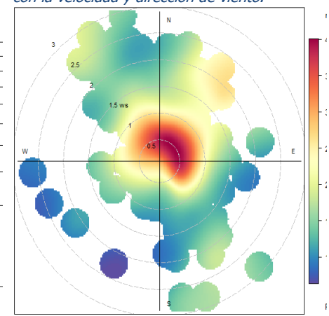
Figura 14: Grafica polar PM10, en relación con la velocidad y dirección de viento.
