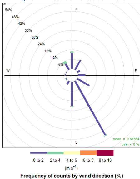
Figura 12: Rosa de vientos abril 2019
