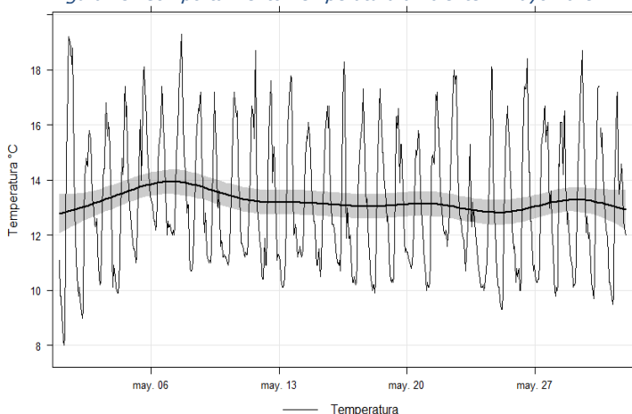
Figura 15: Comportamiento Temperatura ambiente – mayo 2019
