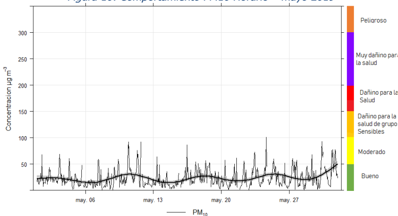
Figura 10: Comportamiento PM10 Horario – mayo 2019
