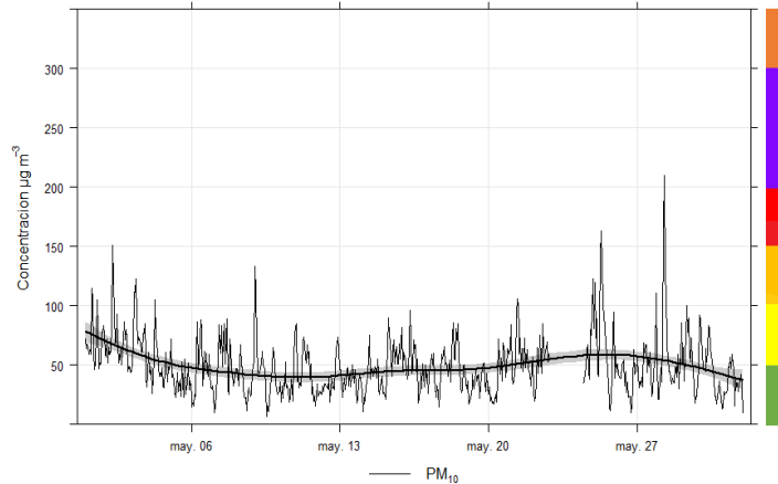
Figura 2: Comportamiento PM10 Horario – mayo 2019
