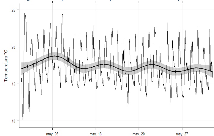
Figura 7: Comportamiento Temperatura ambiente – mayo 2019
