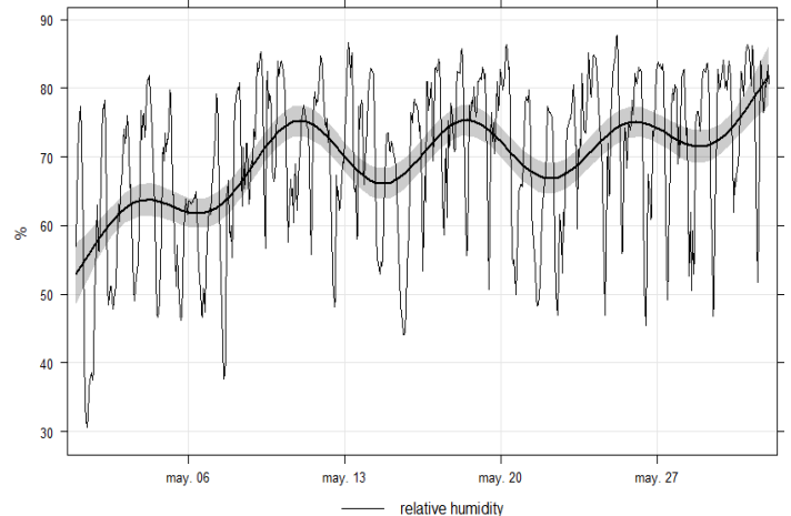
Figura 8: Comportamiento Humedad Relativa – mayo 2019.
