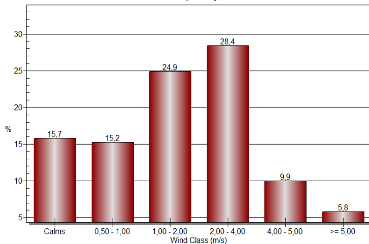
Figura 7. Distribución de velocidad del viento. Octubre 2023. Wind Class Frequency Distribution
