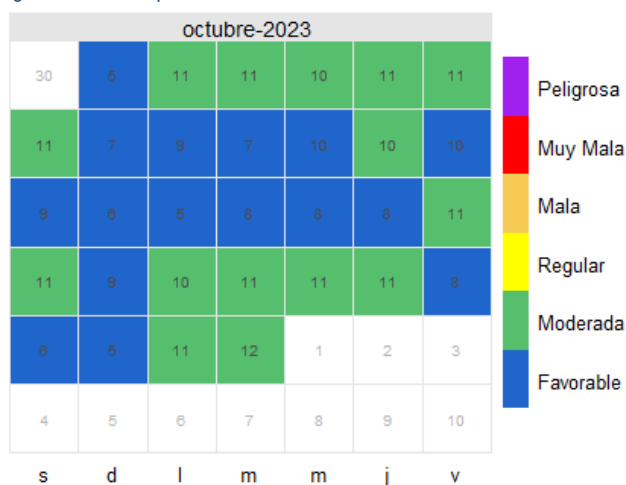
Figura 14. IBOCA pm_{10}
