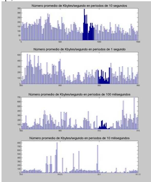
Figure 3. Número promedio de bytes/segundo medidos en intervalos de 0.01, 0.1, 1 y 10 segundos, para una traza real de tráfico en una red LAN (BC_pAug89 [66]).
