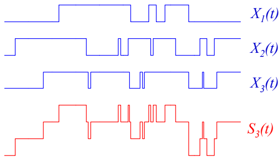
Figura 5. Tráfico agregado proveniente de tres fuentes on/off
