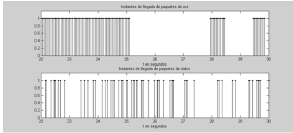
Figura 1. Instantes de Llegada de Paquetes de Voz (MMDP) y Datos (Poisson) en una red LAN
