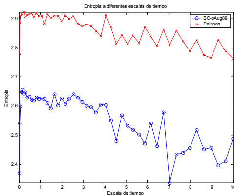
Figura 10. Entropía condicional de los niveles de tráfico a diferentes escalas de tiempo para las dos trazas.
