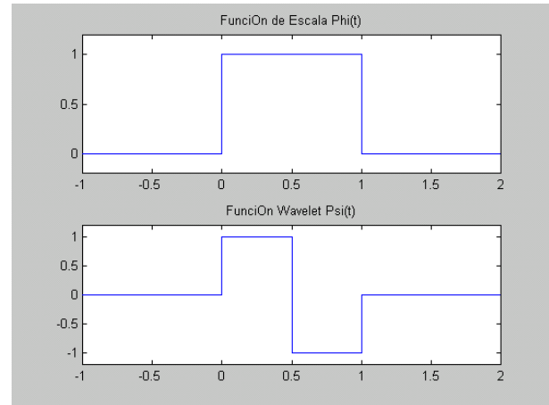
Figura 6. Función de Escala \phi(t) y wavelet \psi(t) para la transformada de Haar.
