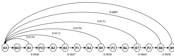
Figura 2. Modelo MMPP para tráfico de video VBR generado por un codificador MPEGII
