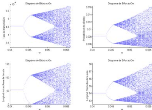
Figura 12. Diagramas de bifurcación para el sistema dinámico de la figura 11.
