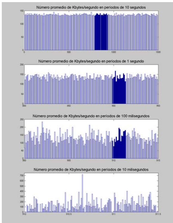
Figure 4. Número promedio de bytes/segundo medidos en intervalos de 0.01, 0.1, 1 y 10 segundos, para una traza de tráfico Poisson.
