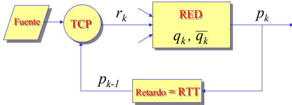
Figura 11. Modelo de sistema dinámico realimentado para una fuente TCP y una cola RED.
