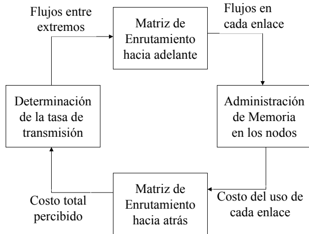
Figura 8. Control de congestión por realimentación mediante ajuste de la tasa de transmisión.
