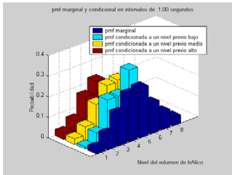
Figura 9. Probabilidad marginal y condicional del nivel del tráfico futuro para las trazas de tráfico de las figuras 3 y 4.
