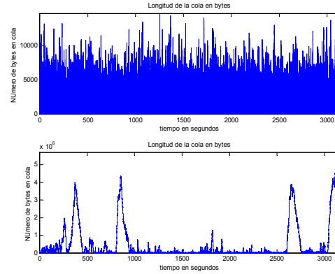
Figura 7. Longitud de la cola en un enlace T1 (a) Con tráfico Poisson (b) Con tráfico fractal.
