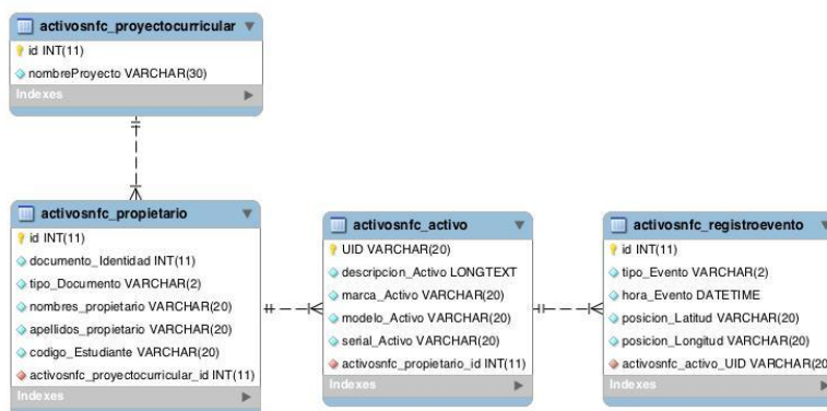
Figura 3: Modelo Entidad Relación
