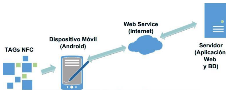
Figura 2: Estructura General del Prototipo
